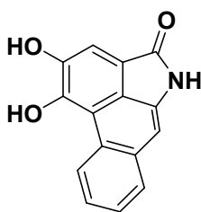
Aristololactame (A-II)
