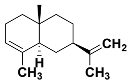
\alpha -selinene
