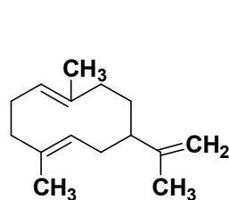
Germacrene-A
