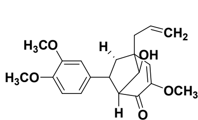
Piperol-A
