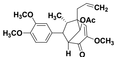
Piperbetol
