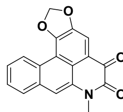
Cepharadione
