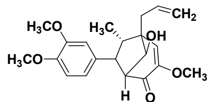
Piperol-B
