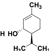
Cis-piperitol
