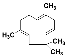
Humulene
