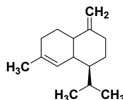
Cadinene
