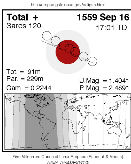
Рис. 1. Лунное затмение 16 сентября 1559 года [9]
