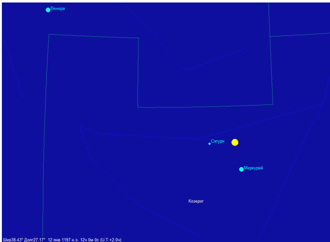
Рис. 2. Положение планет 12 января 1197 года в 12.00.00
