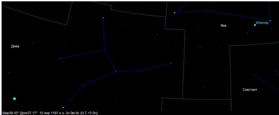
Рис. 1. Положение планет 12 января 1197 года в 03.00.00
