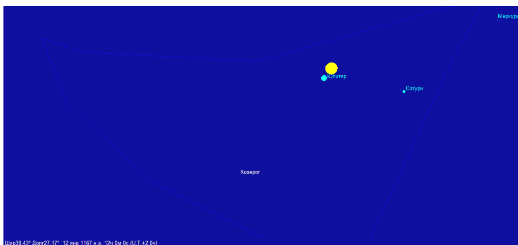
Рис. 3. Положение планет 12 января 1167 года в 12.00.00
