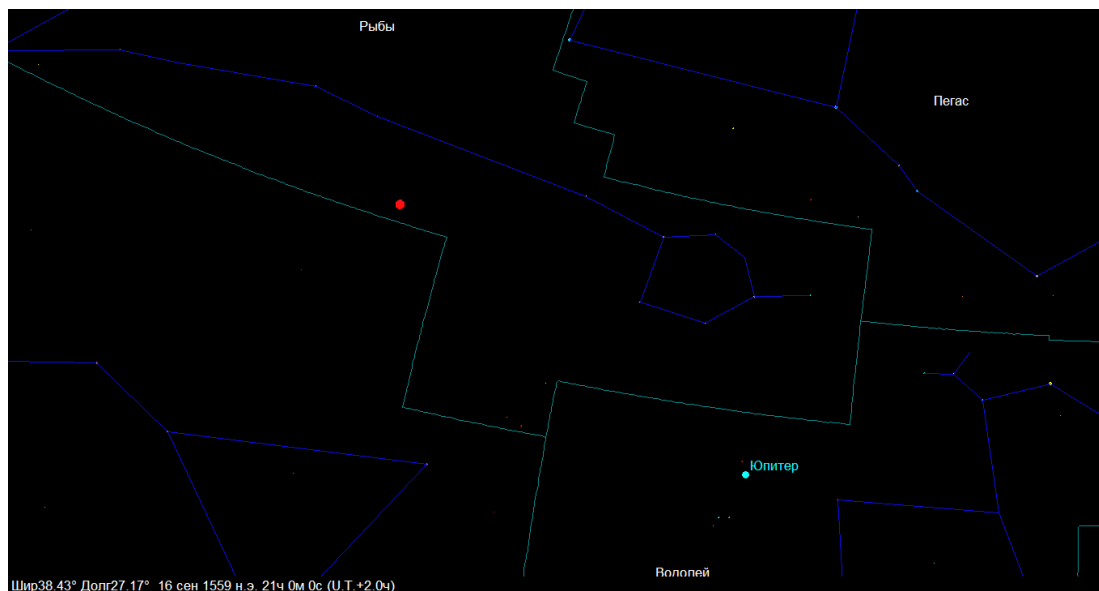
Рис. 2. Положение Луны, затмение окрасило спутник Земли в красный цвет, 16 сентября 1559 года в 21.00.00
