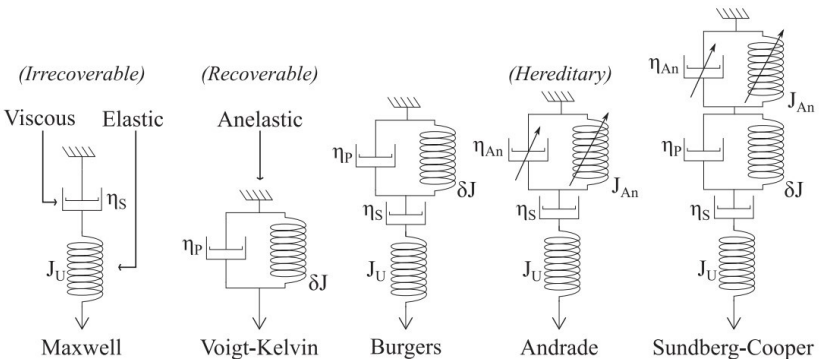
Fig. 1. Rheology
