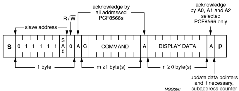
Fig.15 I²C-bus protocol.
