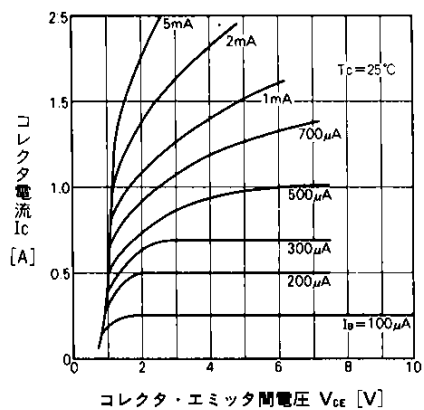
出力特性
