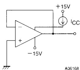
(7) I_{CC}
