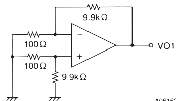
(1) V_{I0} , SVRR
