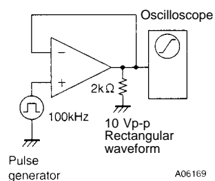
(8) SR
