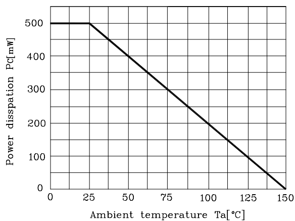
Fig. 1 P_C - T_a
