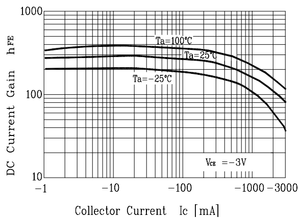
Fig. 5 h_{FE} - I_C
