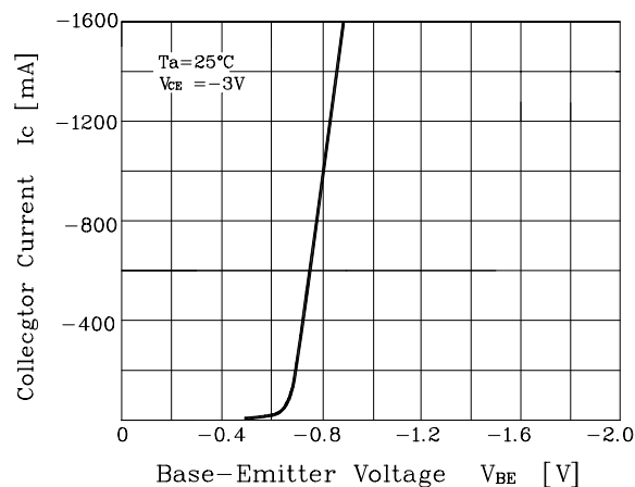
Fig. 2 I_C - V_{BE}
