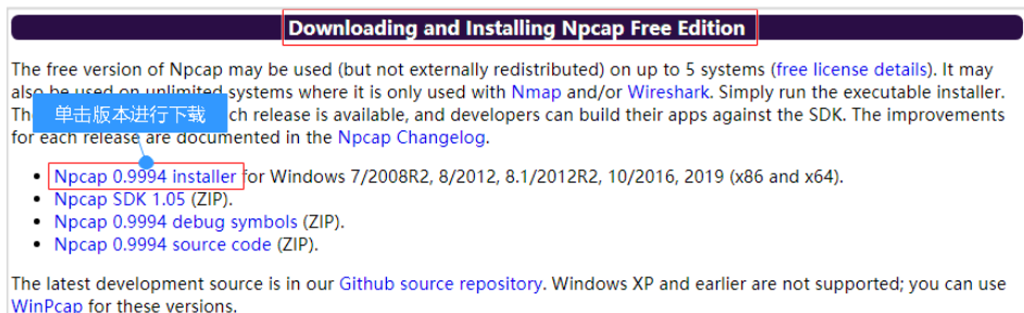
图 4-6 下载 npcap
