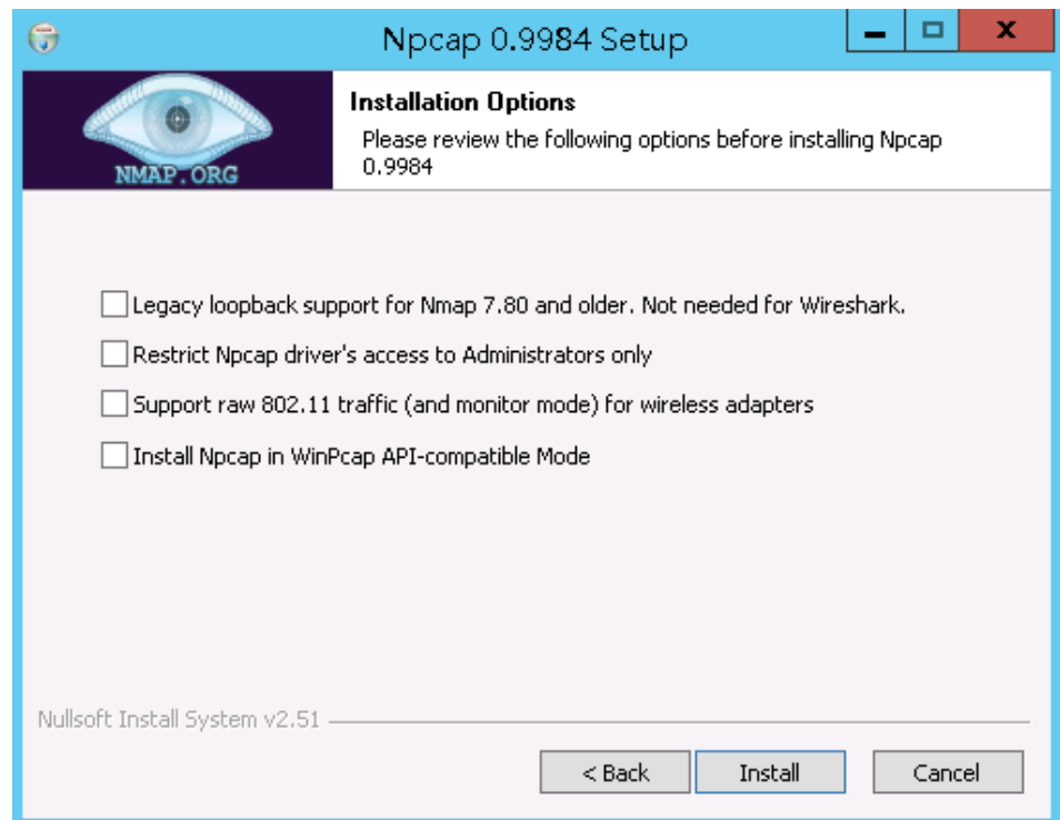
图 4-8 安装 “Npcap”
