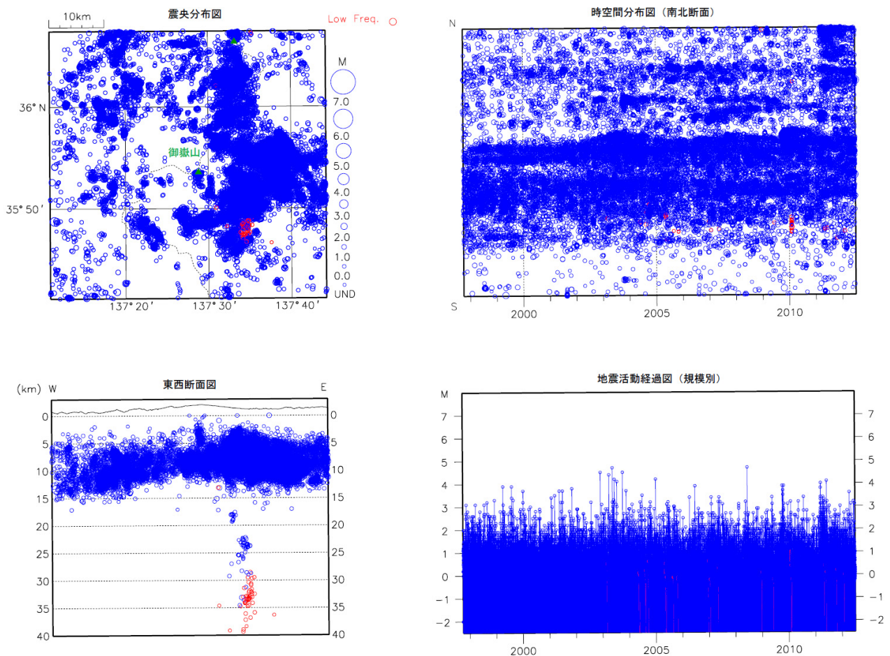
図 53-17 広域地震観測網による浅部の地震活動(青)及び深部低周波地震活動(赤) (1997 年 10 月 1 日～2012 年 6 月 30 日)。
