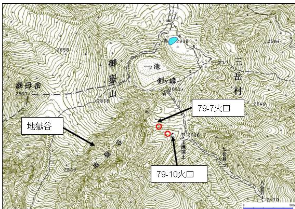
図53-1 火口周辺図.
