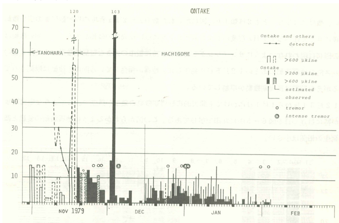
図 53-3 御嶽山における噴火口下の地震日別頻度及び微動の発生（1979 年 11 月～1980 年 4 月）（名古屋大学, 1980）.
