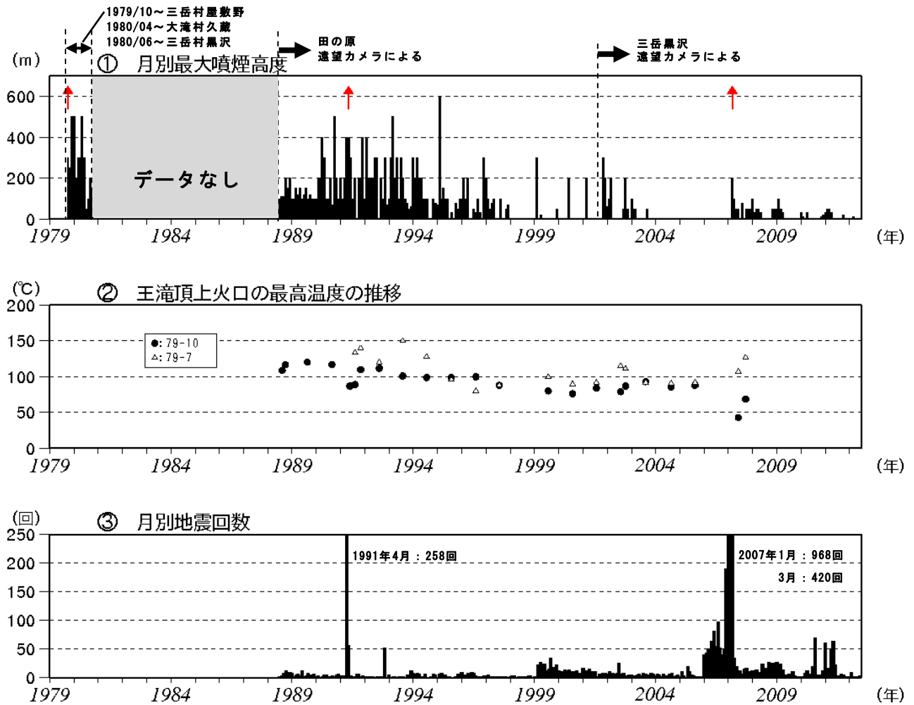
図 53-15 長期の火山活動の推移. ①: 月最大噴煙高度 (1979 年 10 月～2012 年 6 月 30 日), ②: 王滝頂上噴気地帯の温度変化 (1988 年 8 月～2012 年 6 月, サーミスタ温度計による), ③: 月別地震回数グラフ (1988 年 7 月 15 日～2012 年 6 月 30 日).
