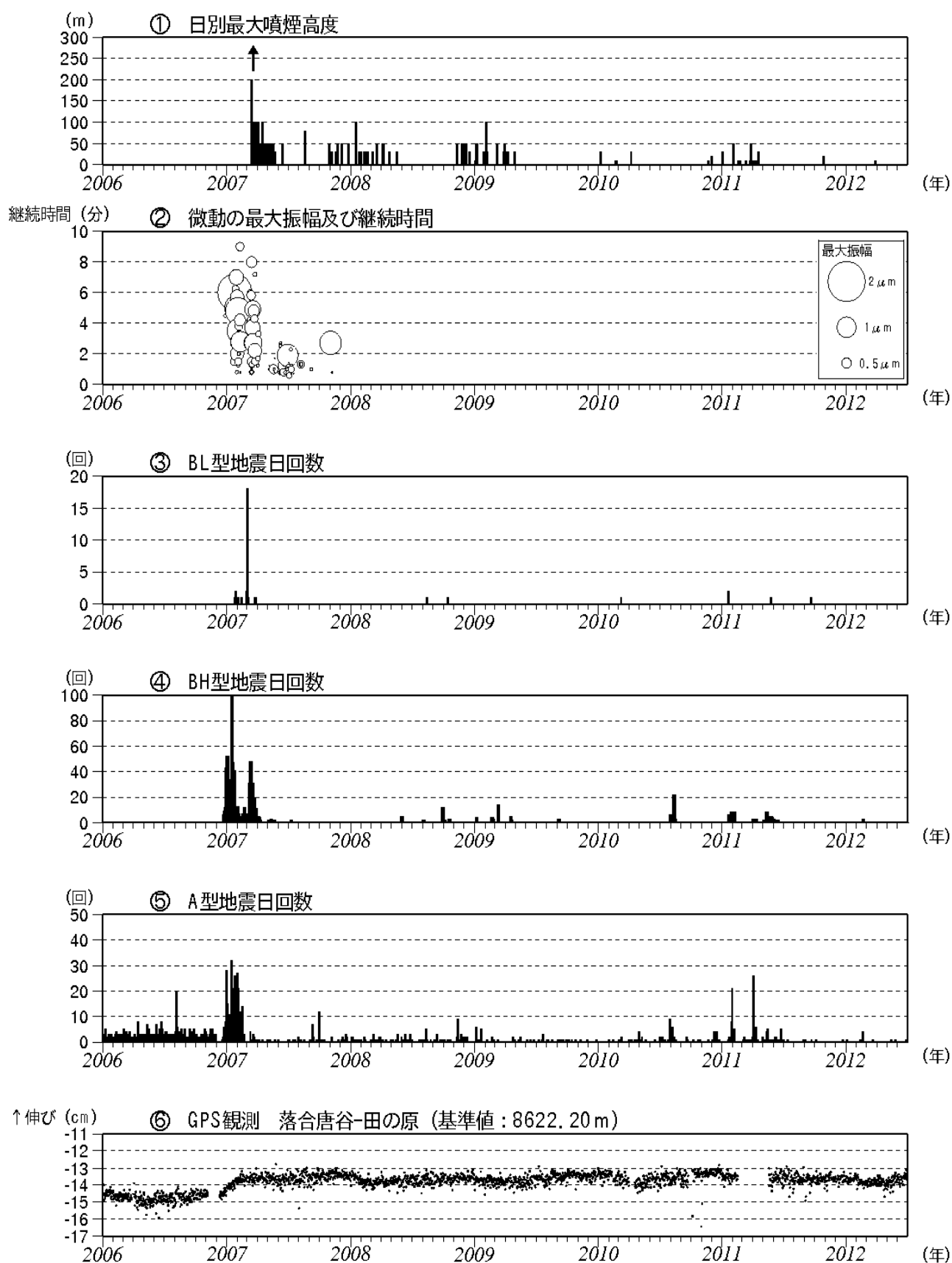
図 53-16 最近の火山活動の推移 (2006 年 1 月 1 日～2012 年 6 月 30 日)。
