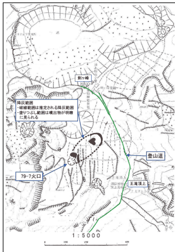
図 53-11 2007 年 5 月 29 日に確認された火山灰の分布図（気象庁，2008）。
