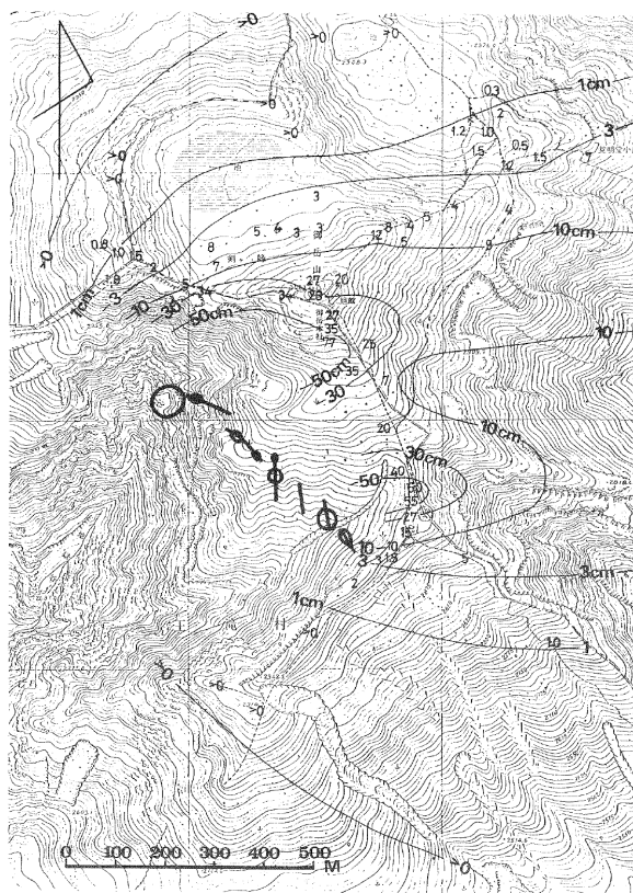
図 53-4 1979 年小火口（割れ目）群と山頂部の火山灰分布（数字は厚さ：cm 単位）（御嶽山 1979 年火山活動および災害の総合的調査研究, 1980）。太線は、10 月 28 日に剣ヶ峰の南斜面に生じた小火口（割れ目），円印は 1979 年 11 月 9 日現在開口の小火口で、全体として北西－南東の配列を示す。
