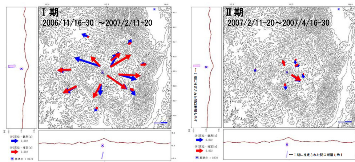
図 53-13 推定された圧力源と変位分布 (気象研究所・気象庁, 2007)。左: 第Ⅰ期 (2006/11/16-30～2007/2/11-20), 右: 第Ⅱ期 (2007/2/11-20～2007/4/16-30)。青矢印: 変位の観測値, 赤矢印: 変位分布の計算値。固定点: GS10270 (豊科)。
