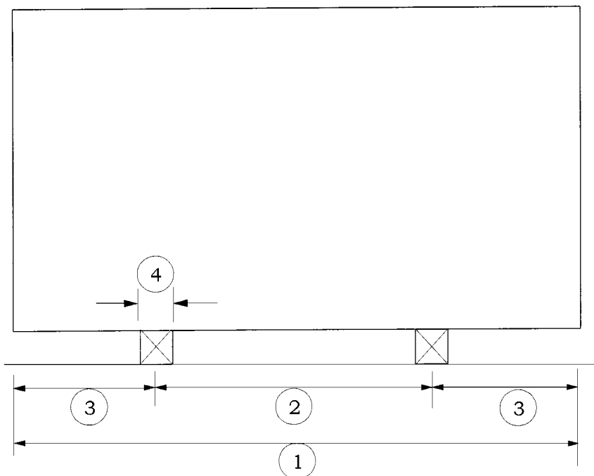
Bild 5: Aufstellbedingungen zum Messen der allgemeinen Verformung
