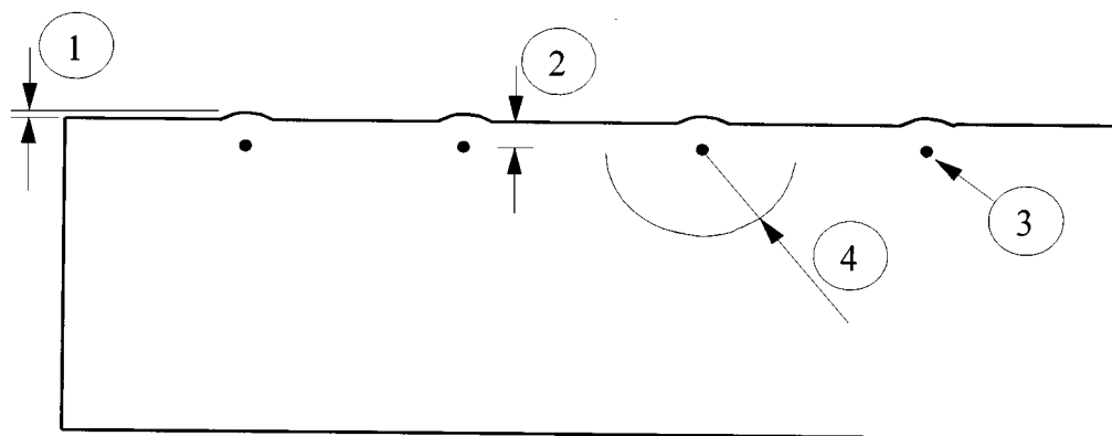
Bild 2: Toleranzen für die Maße von rechteckigen Scheiben
