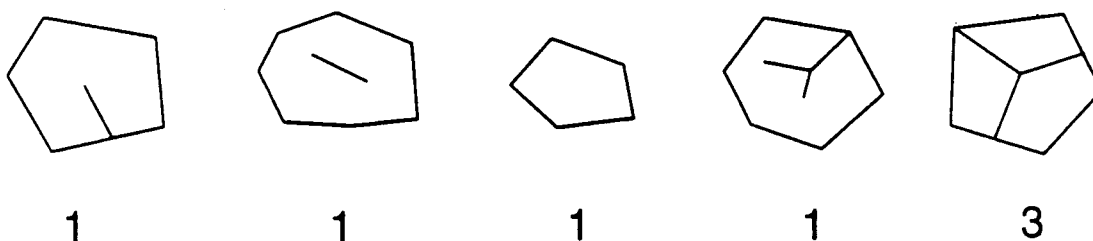
Bild 14: Beispiele anrißfreier Bruchstücke und ihre Bewertung hinsichtlich der Anzahl
