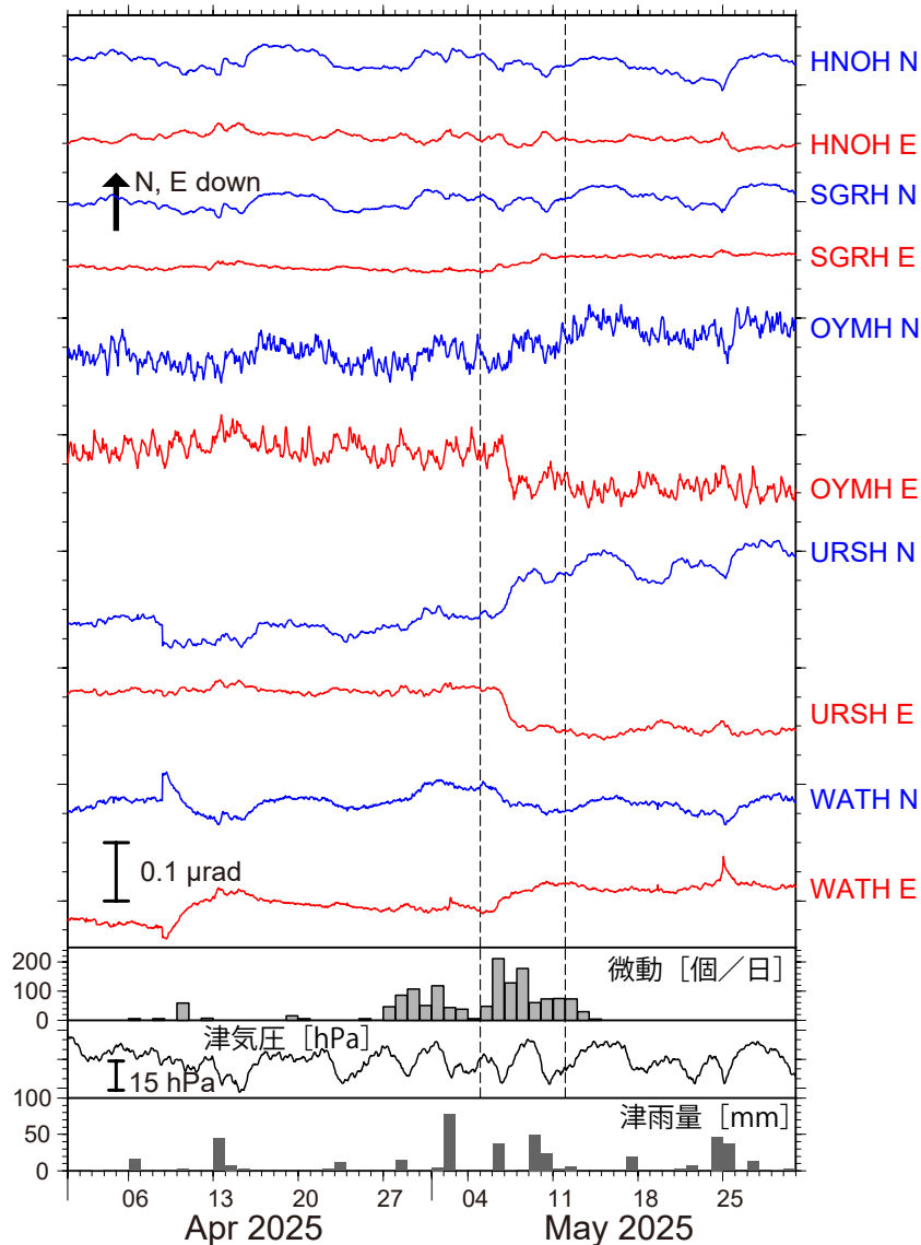
図 1：2025 年 4 月 1 日～5 月 30 日の傾斜時系列。上方向への変化が北・東下がりの傾斜変動を表し、BAYTAP-G により潮汐・気圧応答成分を除去した。5 月 5 日～11 日の傾斜変化ベクトルを図 2 に示す。紀伊半島北部～愛知県西部での微動活動度・気象庁津観測点の気圧・雨量をあわせて示す。
