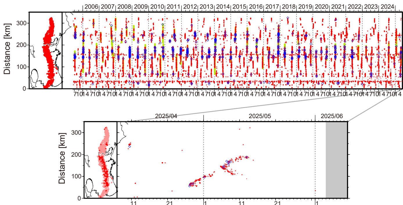
図 1. 紀伊半島・東海地域における 2005 年 6 月～2025 年 6 月 3 日までの深部低周波微動の時空間分布（上図）。赤丸はエンベロープ相関・振幅ハイブリッド法 (Maeda and Obara, 2009) およびクラスタ処理 (Obara et al., 2010) によって 1 時間毎に自動処理された微動分布の重心である。青菱形は周期 20 秒に卓越する超低周波地震 (Ito et al., 2007) である。黄緑色の太線はこれまでに検出された短期的スロースリップイベント (SSE) を示す。下図は 2025 年 5 月を中心とした期間の拡大図である。4 月 27 日～5 月 14 日頃には、奈良・和歌山県境付近から三重県北部において活発な微動活動がみられた。この活動は奈良県南部で開始した後、北東方向への活動域の移動が 5 月 4 日頃までみられた。5 月 5 日 17:05 頃に三重県北部の深さ約 19 km で発生した M2.9 の地震 (Hi-net 暫定値) 後の 17:10 過ぎからは三重県中部で活動が活発化し、北東および南西方向への活動域の移動がみられた。南西方向の活動は奈良・三重県境付近まで達し、11 日頃まで活動がみられた。北東方向の活動は三重県北部に達し、14 日頃まで活動がみられた。この活動に際し、傾斜変動から短期的 SSE の断層モデルも推定されている。
