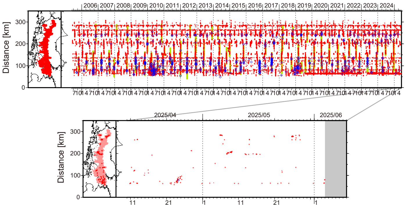
図 1. 四国における 2005 年 6 月～2025 年 6 月 3 日までの深部低周波微動の時空間分布（上図）。赤丸はエンベロープ相関・振幅ハイブリッド法 (Maeda and Obara, 2009) およびクラスター処理 (Obara et al., 2010) によって 1 時間毎に自動処理された微動分布の重心である。青菱形は周期 20 秒に卓越する超低周波地震 (Ito et al., 2007) である。黄緑色太線は、これまでに検出された短期的スロースリップイベント (SSE) を示す。下図は 2025 年 5 月を中心とした期間の拡大図である。5 月以降の期間について、顕著な活動はとくにみられなかったものの、愛媛県東部において、5 月 7～9 日頃に小規模な活動が、5 月 12～13 日および 15～16 日頃にごく小規模な活動がみられた。5 月 25～28 日頃には徳島県中部から香川・徳島県境付近において、小規模な活動がみられた。5 月 5～6 日には香川県付近、5 月 13～14 日頃には香川・徳島県境付近において、それぞれごく小規模な活動がみられた。
