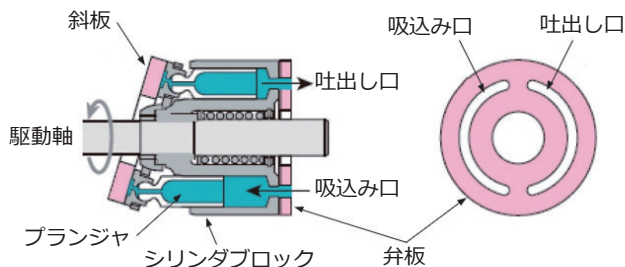
図2-7 プランジャポンプ
