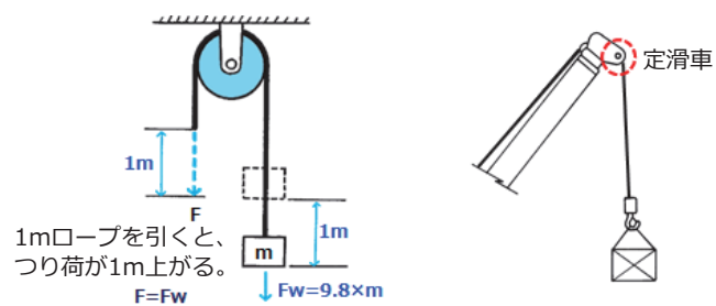
図3-14 定滑車
