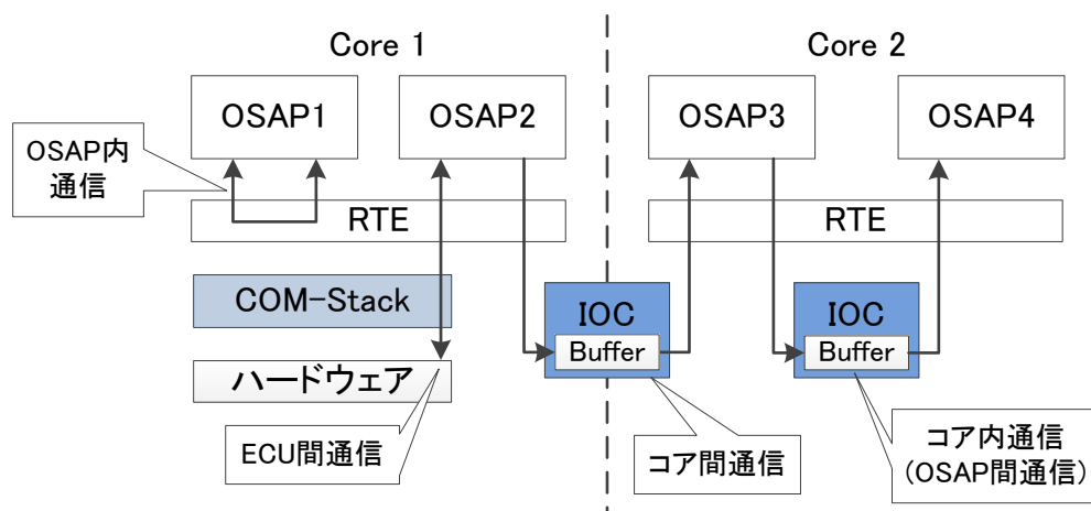
図 2-54 IOC によるデータ通信
