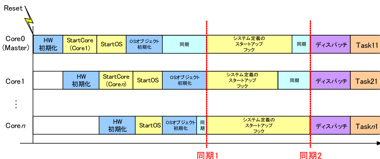
図 2-52 マルチコアシステムの初期化手順
