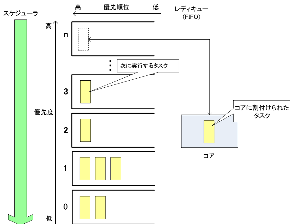
図 2-10 スケジューラによる実行タスクの検索
