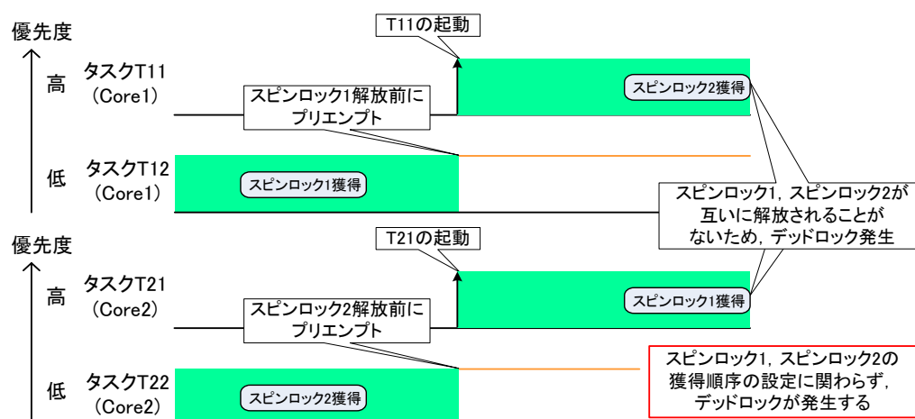
図 2-61 スピンロックによるデッドロックの例 3
