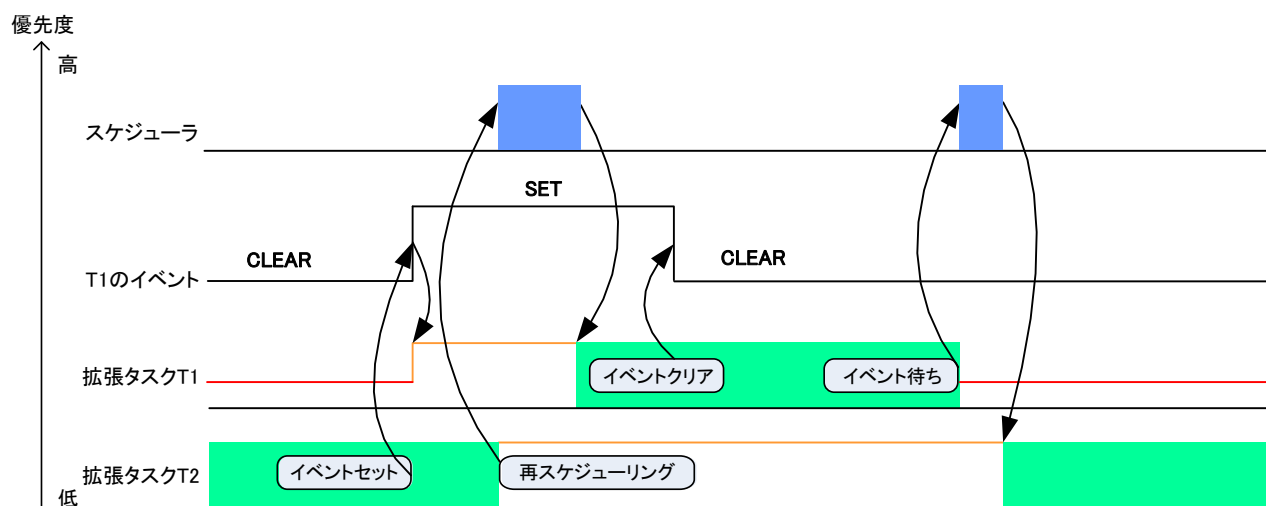
図 2-18 ノンプリエンプティブタスクの同期例
