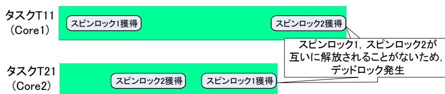
図 2-59 スピンロックによるデッドロックの例 2
