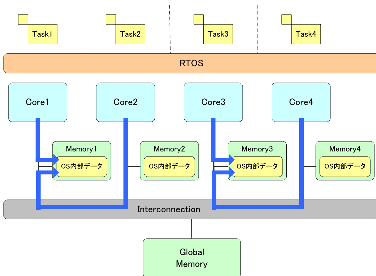
図 2-7 直接操作法によるコア間システムサービス実装
