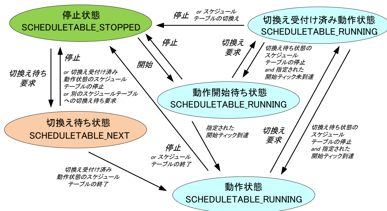
図 2-25 同期なしスケジュールテーブルの状態遷移図
