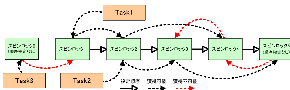
図 2-60 スピンロックの獲得可否
