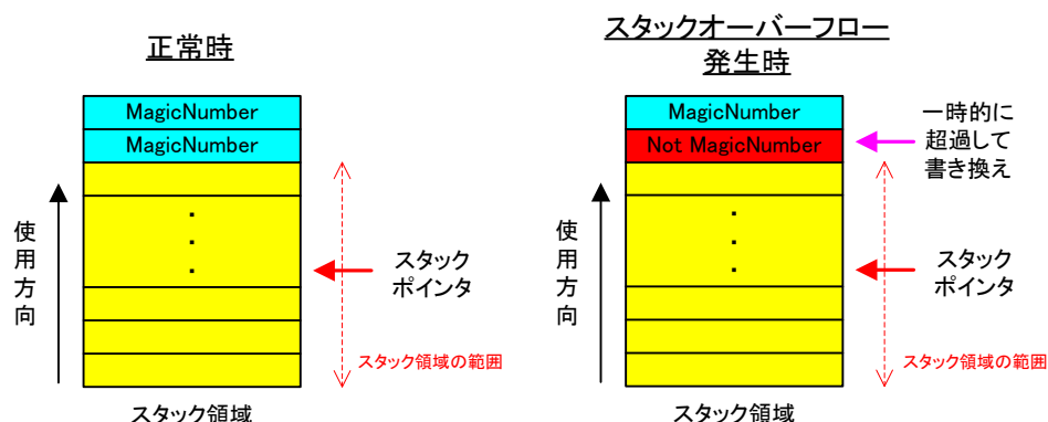
図 2-35 マジックナンバーチェック方式
