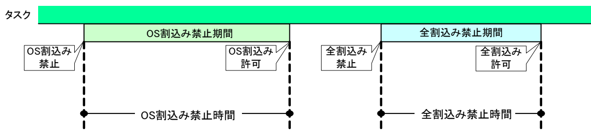
図 2-44 割込み禁止時間
