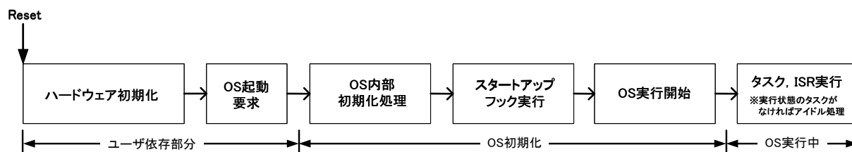
図 2-51 システム初期化シーケンス
