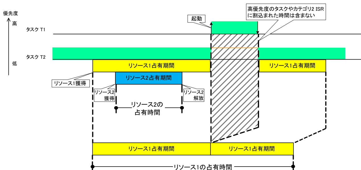
図 2-43 リソース占有時間
