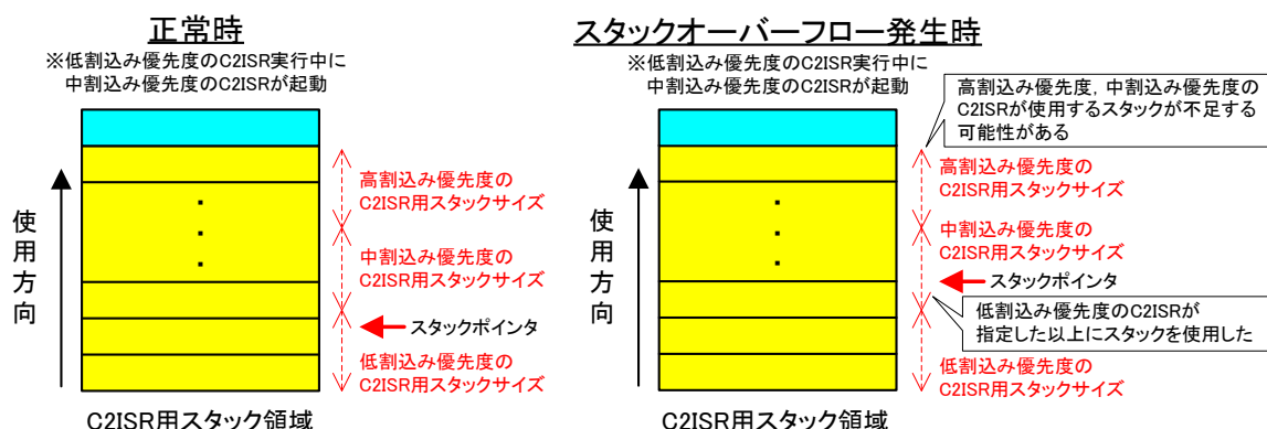
図 2-36 スタック残量チェック方式
