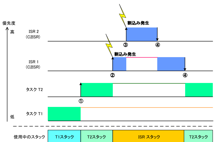
図 2-37 ATK2 におけるスタックモニタリングのタイミング
