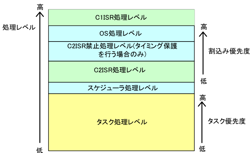
図 2-2 処理レベルと優先度
