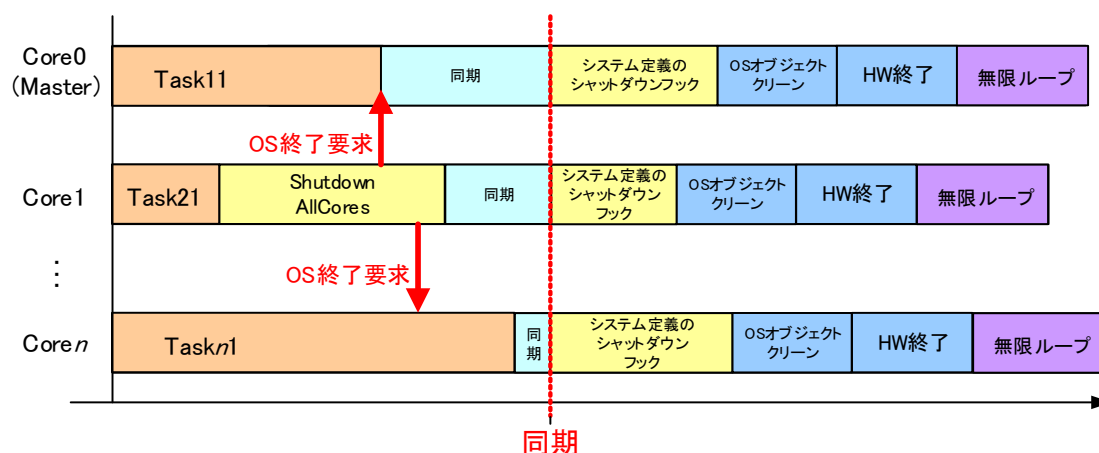
図 2-53 同期 OS シャットダウンによるマルチコアシステム終了手順
