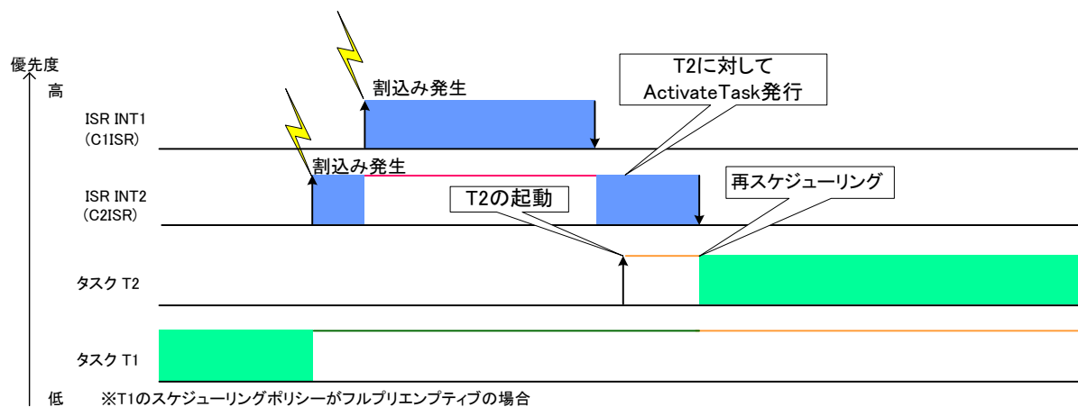
図 2-15 ISR 終了後の再スケジューリング動作の例
