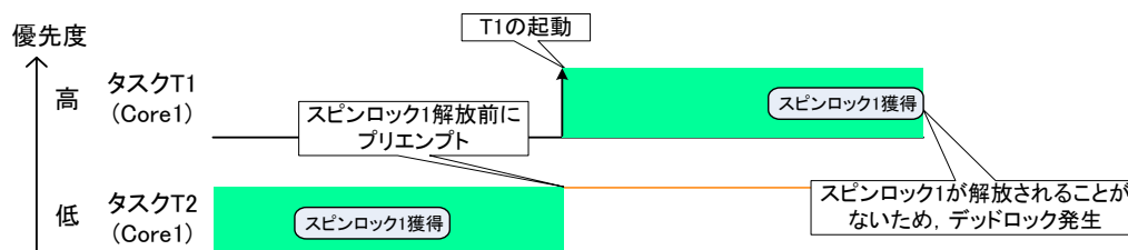
図 2-58 スピンロックによるデッドロックの例 1
