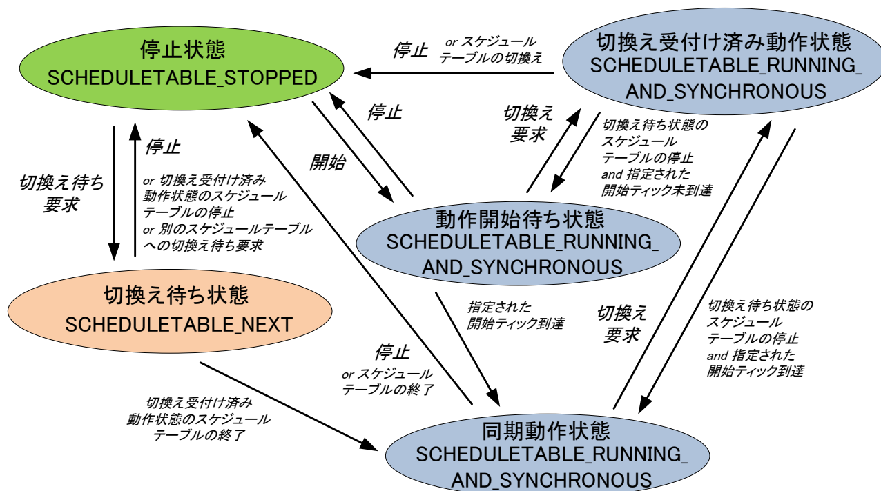
図 2-26 暗黙同期スケジュールテーブルの状態遷移図
