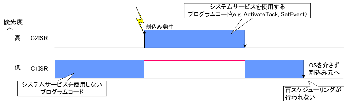
図 2-16 C1ISR に C2ISR が割込んだ場合の問題点
