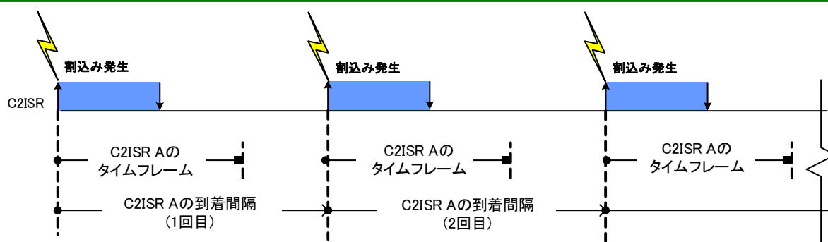
図 2-42 C2ISR 到着間隔
