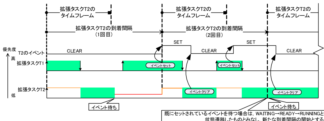
図 2-41 拡張タスクの到着間隔
