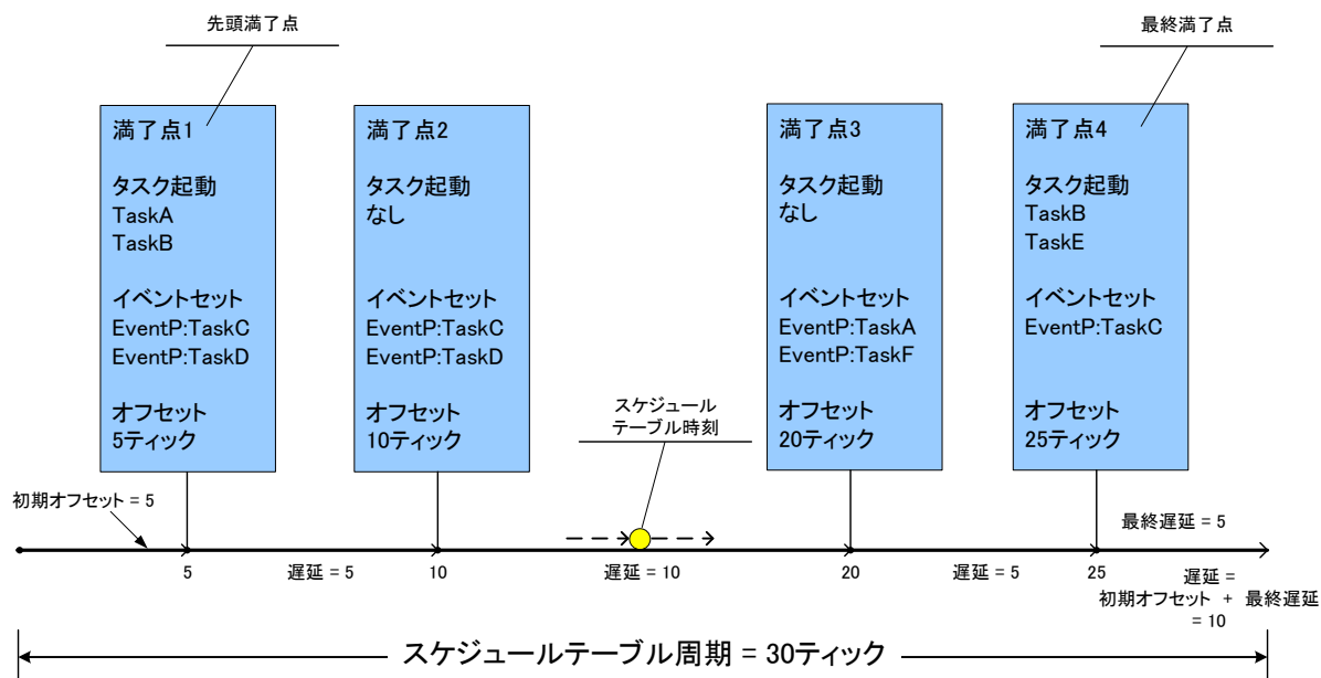
図 2-24 スケジュールテーブルの構成
