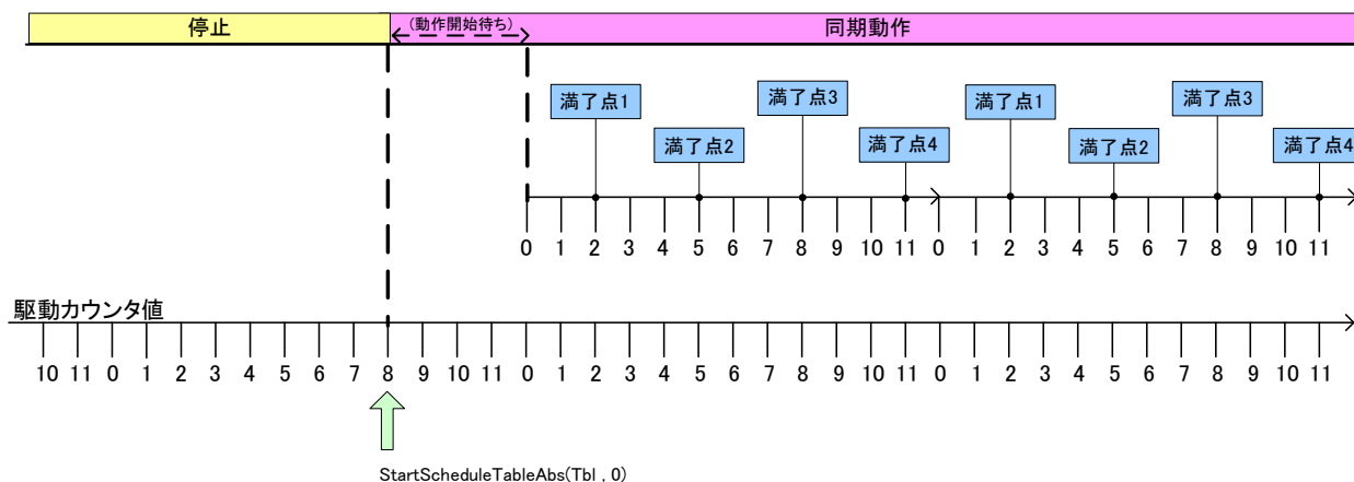
図 2-30 暗黙同期スケジュールテーブルの動作
