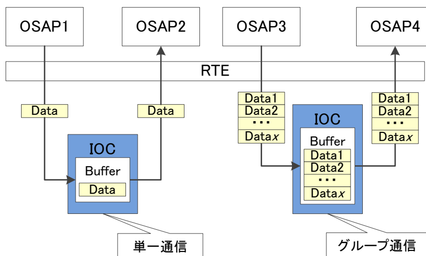
図 2-57 単一通信とグループ通信
