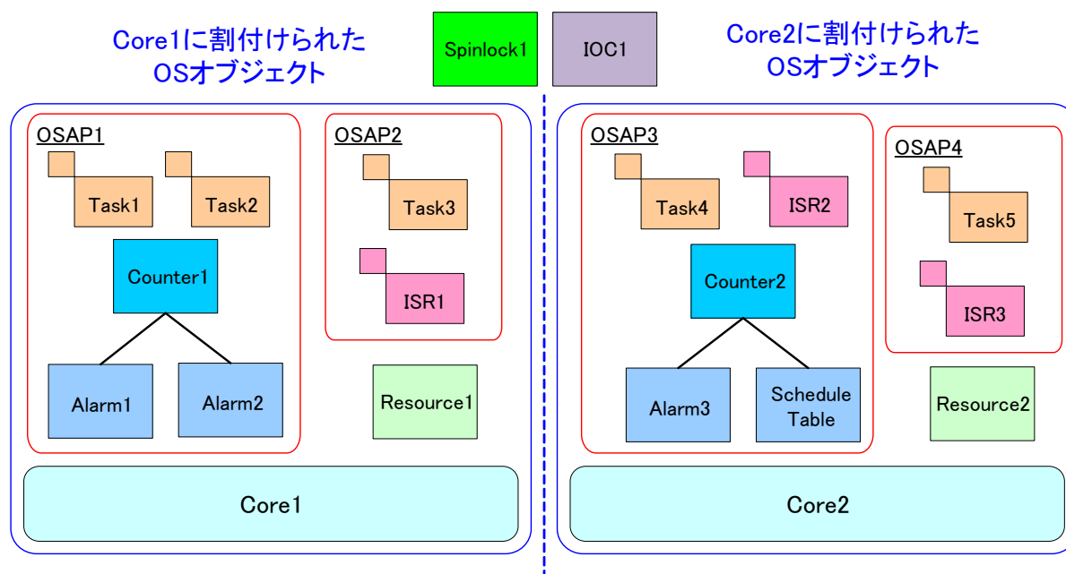
図 2-5 OS オブジェクトのコア割付け
