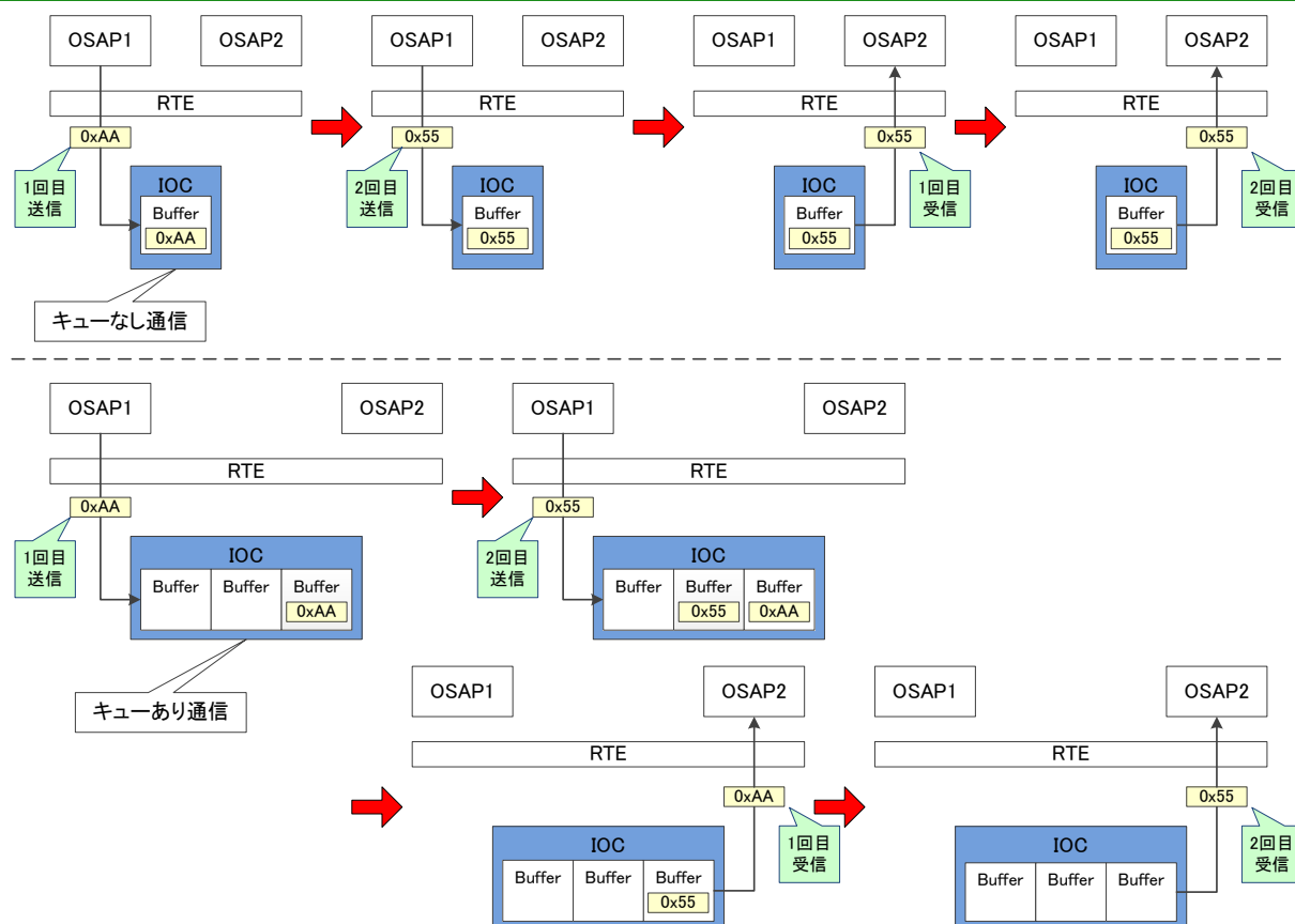
図 2-56 キューなし通信とキューあり通信
