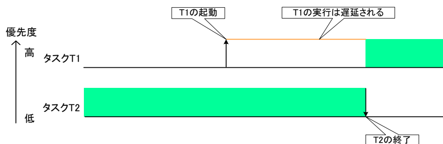
図 2-12 ノンプリエンプティブスケジューリングの例
