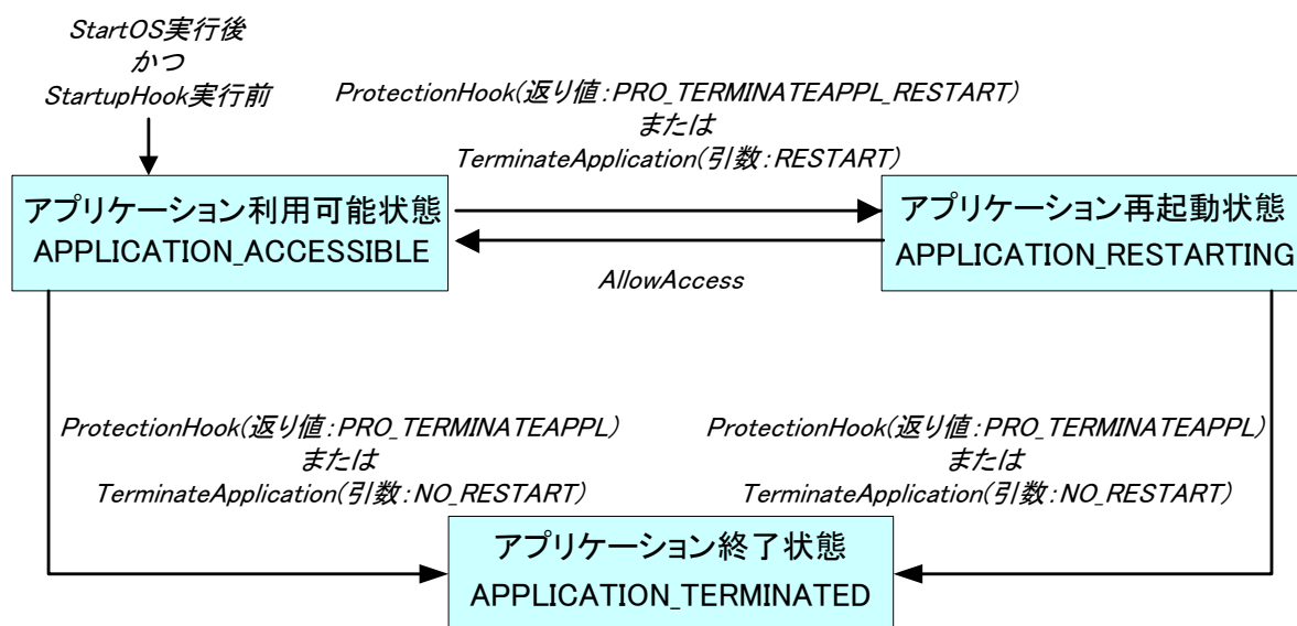
図 2-46 OSAP の状態遷移図
