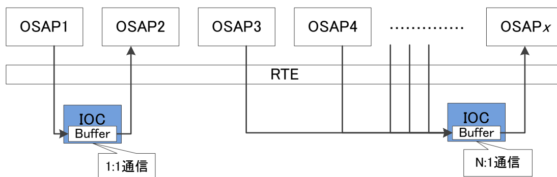
図 2-55 1:1 通信と N:1 通信
