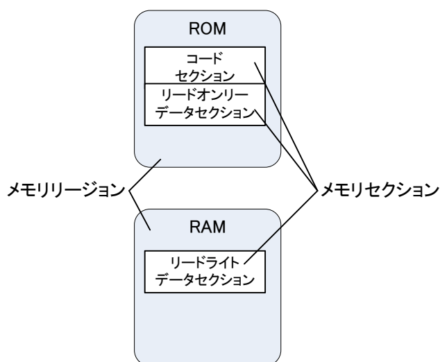
図 2-49 メモリアリジョンとセクションの関係
