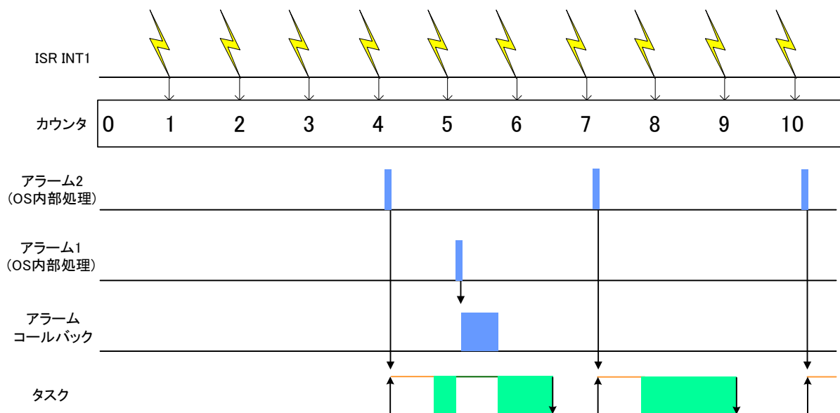
図 2-23 アラームの動作例
