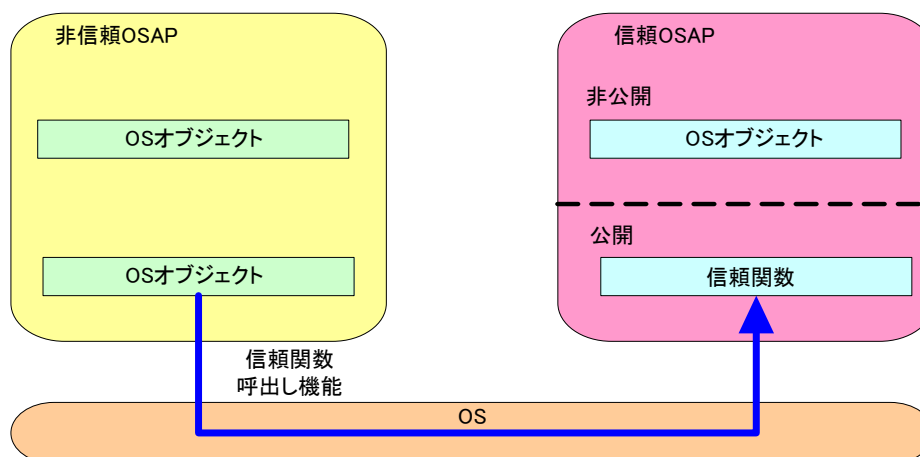
図 2-48 信頼関数を呼び出すための機能
