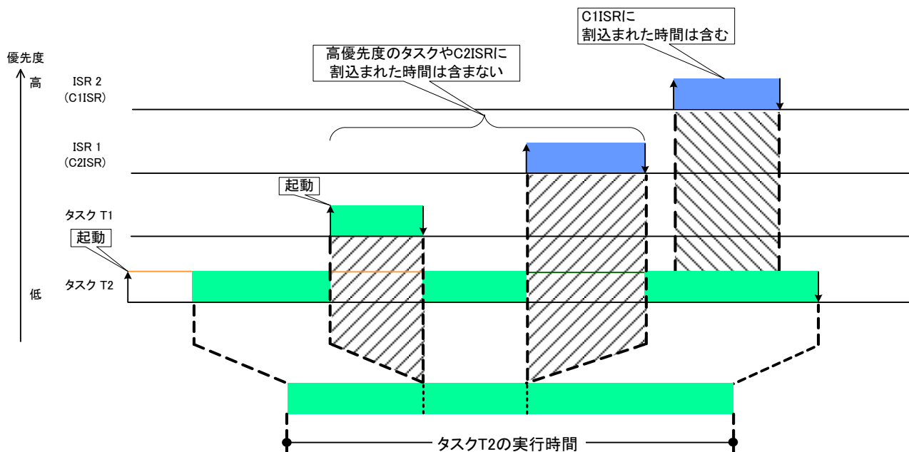
図 2-38 タスク実行時間
