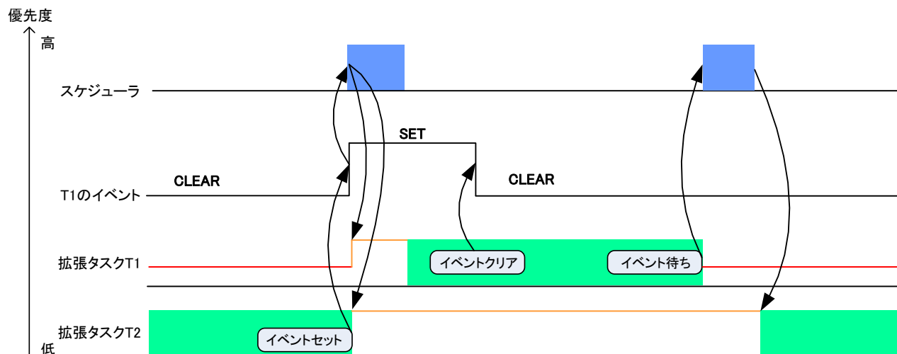
図 2-17 プリエンプティブタスクの同期例
