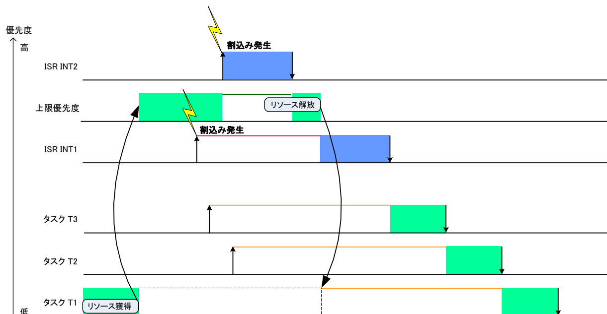
図 2-20 タスク-C2ISR 間の排他例
