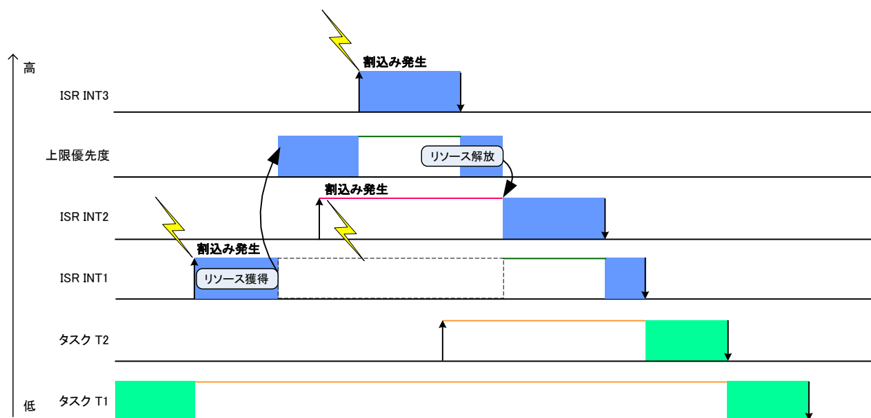
図 2-21 C2ISR－C2ISR 間の排他例
