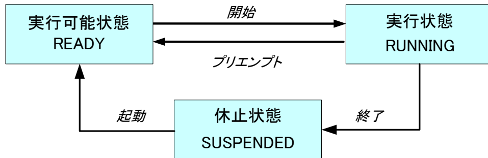
図 2-8 基本タスクのタスク状態遷移図
