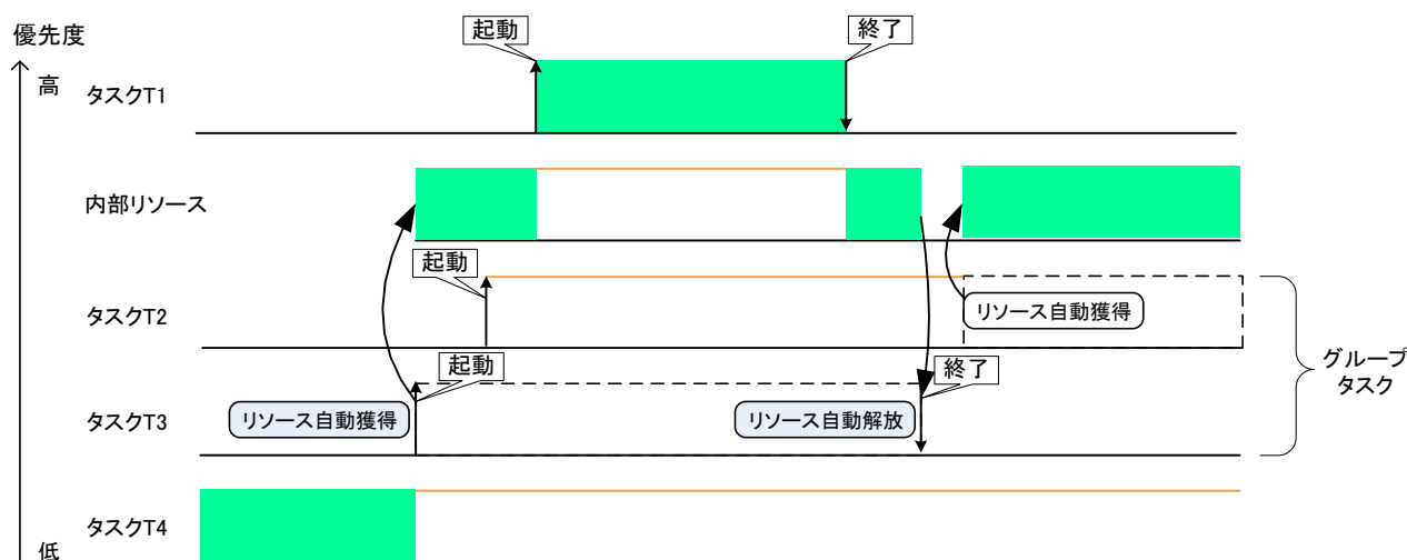
図 2-14 グループタスクの動作例
