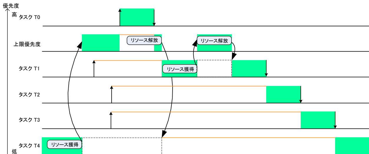
図 2-19 リソースによるタスク間の排他例
