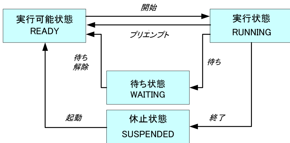
図 2-9 拡張タスクのタスク状態遷移図
