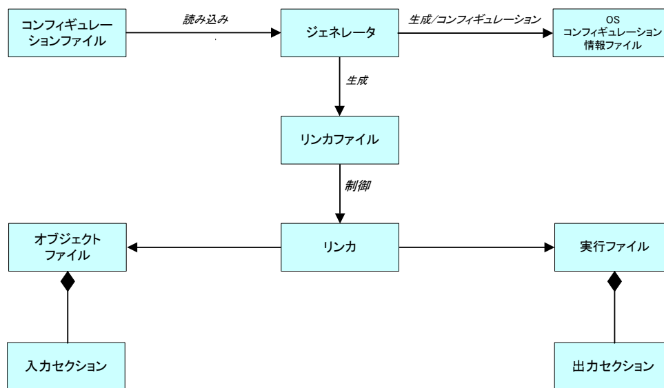
図 2-62 コンフィギュレーション手順
