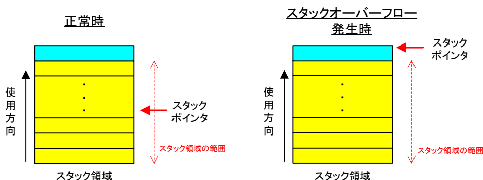
図 2-34 スタックポインタチェック方式
