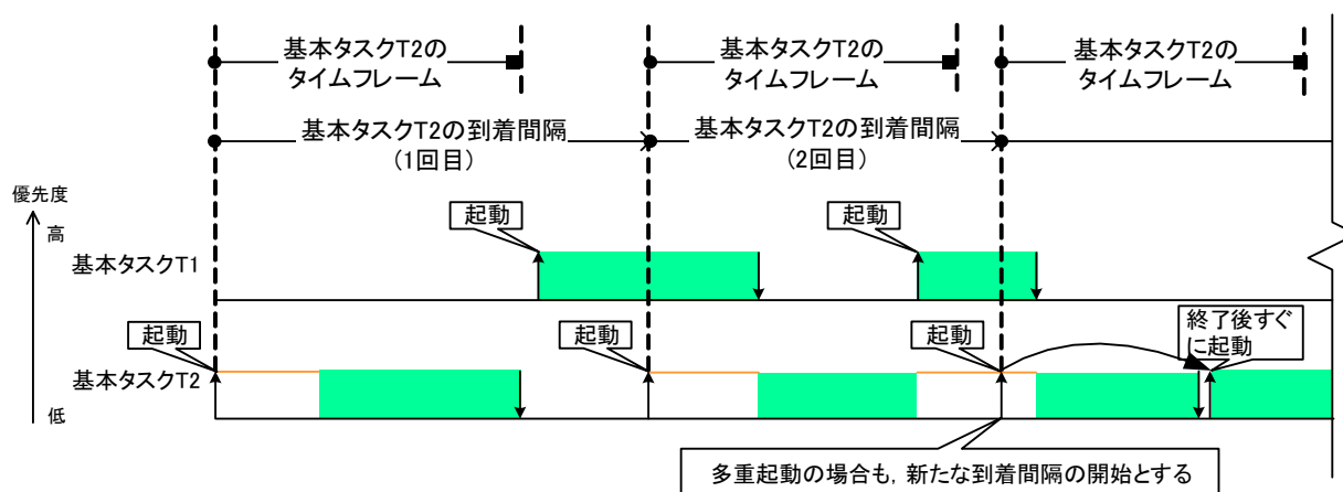
図 2-40 基本タスクの到着間隔
