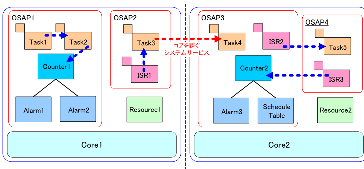
図 2-6 コアを跨ぐシステムサービス
