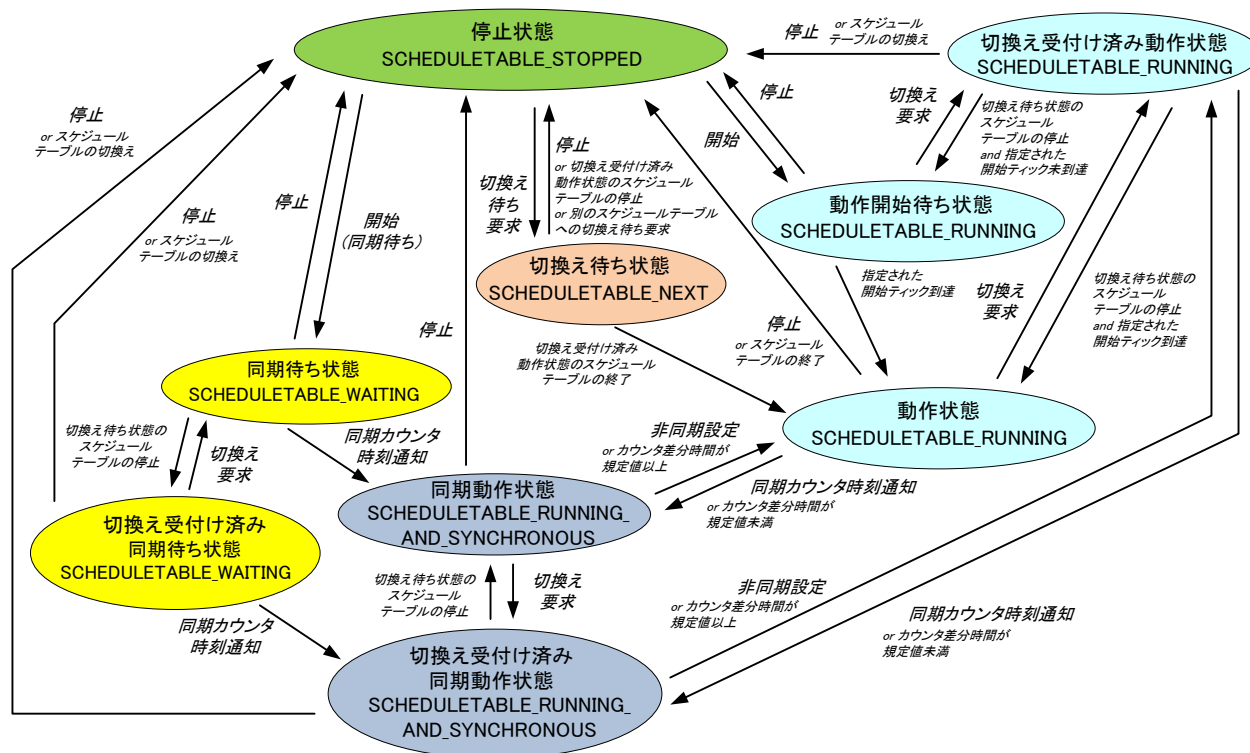
図 2-27 明示同期スケジュールテーブルの状態遷移図
