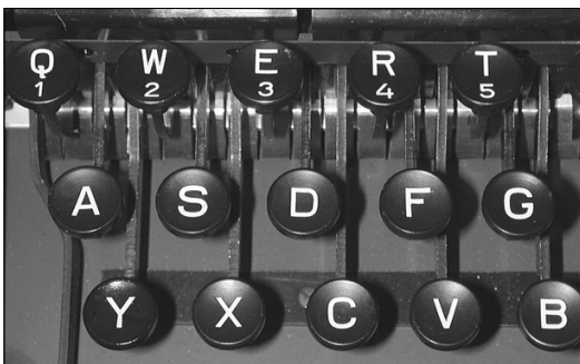
88 Die obere Tastenreihe ist bei der Nema mit Zahlen und Buchstaben beschriftet. [AUT]
