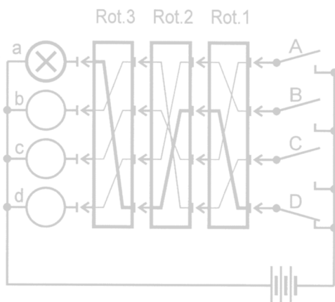
37 Die Anordnung mit drei Rotoren. [AUT]
