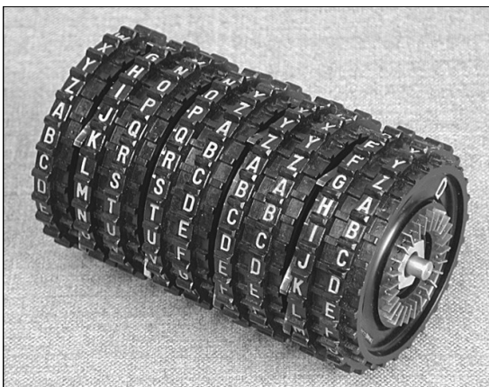
54 Das Herz der Nema: Das Rotor- oder Walzenpaket. Die rote 10. Walze verbleibt in der Maschine. [AUT]
