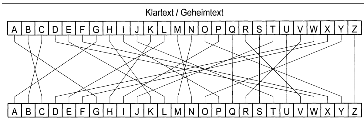
41 Eine involutorische Umsetzung. [AUT]
