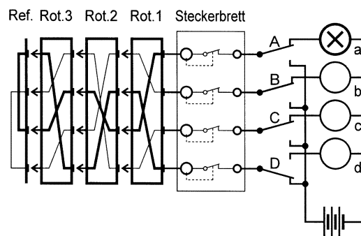
43 Die Enigma: Drei Rotoren und der Reflektor; zusätzlich ist ein Steckerbrett vorhanden. [AUT]
