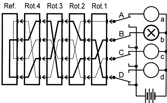
53 Kryptologisches Schema der Nema. Der drehbare Reflektor bekommt die Eigenschaft eines Rotors, ein Steckerbrett fehlt. Die fünf Fortschaltwalzen sind hier nicht gezeichnet, sie tragen nicht direkt zur Permutierung bei. [AUT]
