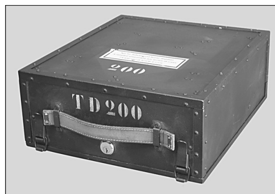
50 Ansicht der geschlossenen Nema, ein schwarzer Koffer mit einem Gewicht von fast 11 kg und den Abmessungen: 33 x 38 x 15 cm. [AUT]
