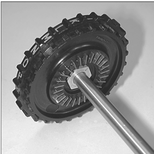
69 Die Umkehrwalze mit fest angebauter Achse. [AUT]
