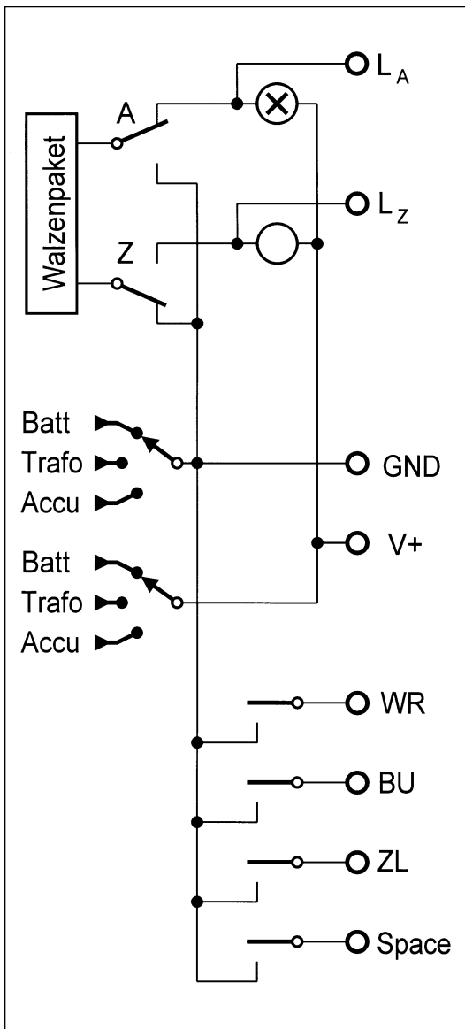
153 Die Interne Verdrahtung und die Steckerbelegung bei der Nema, vereinfacht dargestellt. [AUT]
