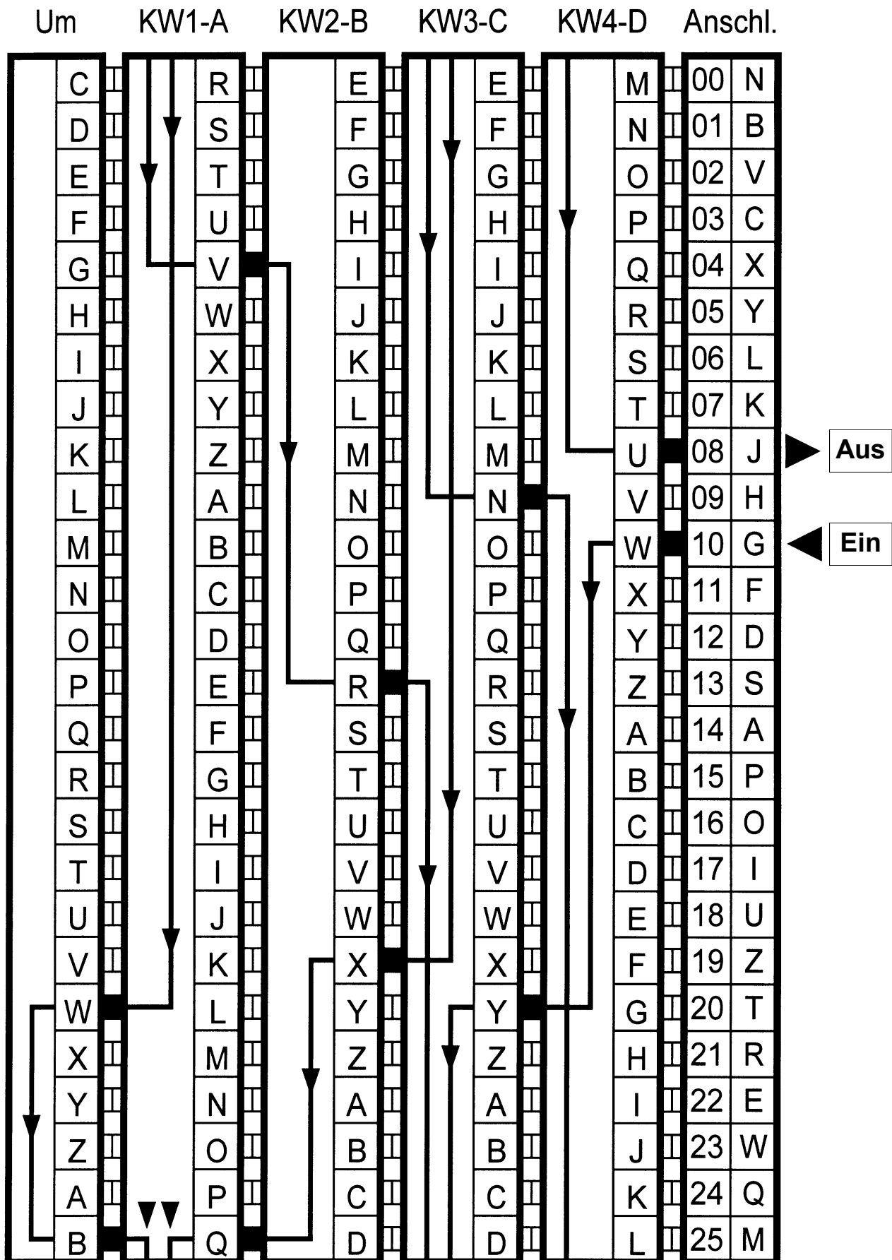
145 Das Berechnungsschema nach Abb. 143 ist hier in grafischer Form dargestellt. [AUT]
