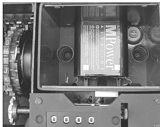
63 Das Batteriefach. An Stelle der grossen Originalbatterie kann eine 4,5-Volt-Taschenlampen-Batterie eingesetzt werden. Ob "auf dem Bauch" oder "auf dem Rücken" liegend ist nicht von Bedeutung. Eine Aussparung (hinten) und eine Feder (vorn) fixieren die Batterie. [AUT]
