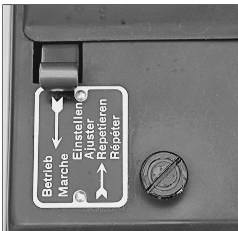
71 Der rote Hebel, rechts daneben eine der beiden Schrauben mit dem roten Ring. [AUT]
