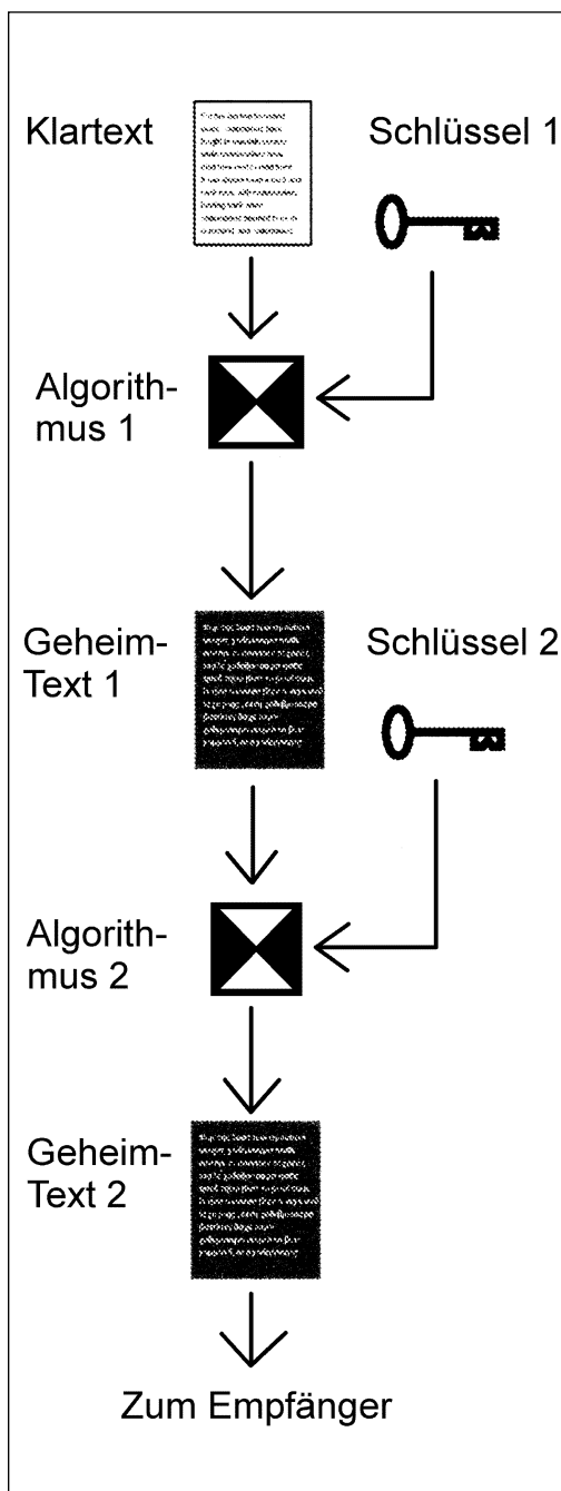
98 Das Prinzip der Mehrfachverschlüsselung. [16] [AUT]
