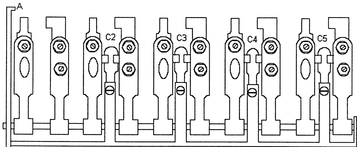
126 Die Zungensteuerung. Der Hebel 'A' (er wird gesteuert von der rechten Nockenscheibe an der roten Walze) drückt über ein Gestänge und die Platten C2, C3, C4 und C5 die Zungen von den Walzen weg, der Vorschub stösst dann ins Leere. Zwischen den Platten und dem Gestänge sind die vier Schrauben sichtbar für die Einstellung der Fortschaltmechanik. [17]
