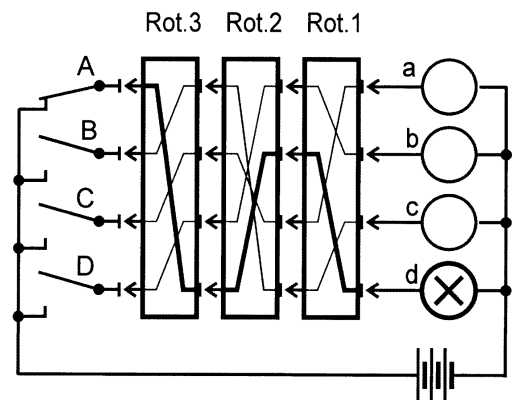
39 Zum Dechiffrieren könnte man Tastatur und Lampenfeld miteinander vertauschen. [AUT]
