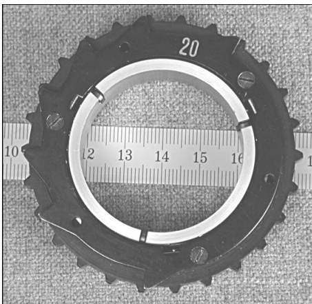
119 Fortschaltwalze mit der Nocken- oder Zahnscheibe Nr. 20 versehen. [AUT]
