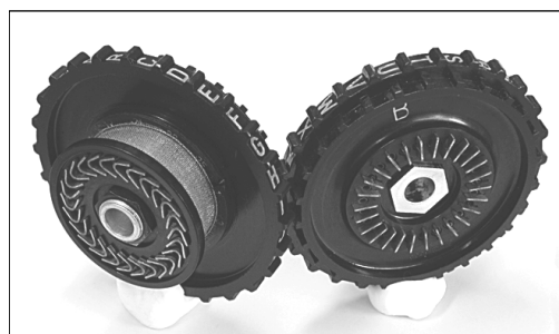
35 Zwei reale Rotoren aus der Chiffriermaschine Nema. [AUT]
