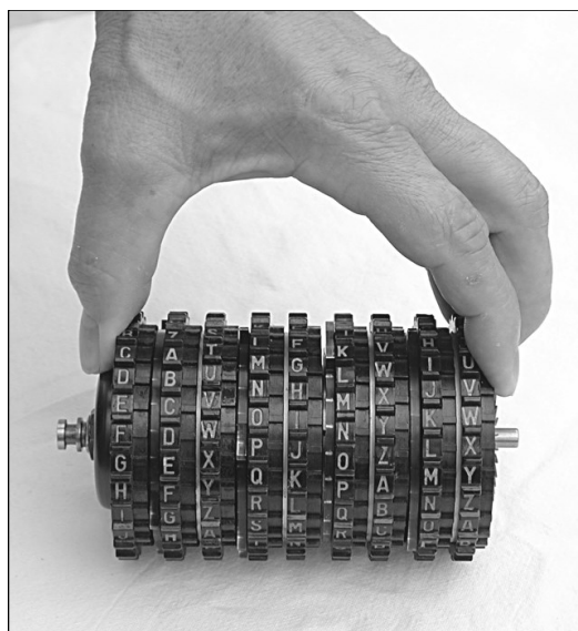
64 Für den Ein- und Ausbau wird das Walzenpaket so gefasst und leicht zusammengepresst. [AUT]
