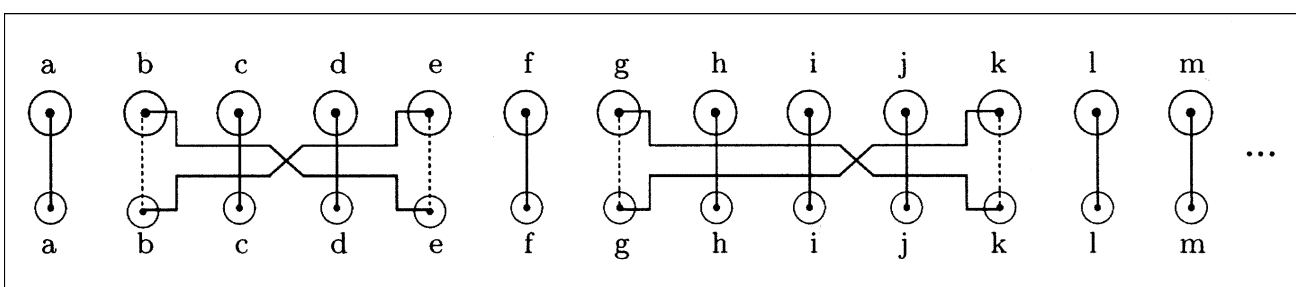
46 Das Prinzip des Steckerbretts bei der Enigma. Zwei Doppelsteckerpaare sind verwendet, das erste von 'b' nach 'e', das andere von 'g' nach 'k'. [5]
