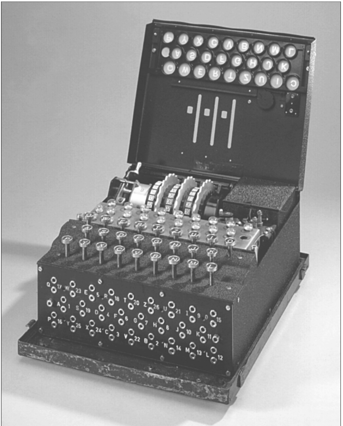
47 Eine Drei-Rotoren-Enigma im Metallkoffer, die Lampenabdeckung ist hochgeklappt. Es existieren verschiedene Ausführungen, meist jedoch solche mit Holzgehäuse. [16]
