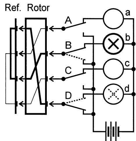
40 Der Reflektor des Deutschen Willi Korn. Die gestrichelten Linien zeigen die Verhältnisse beim Dechiffrieren. [AUT]
