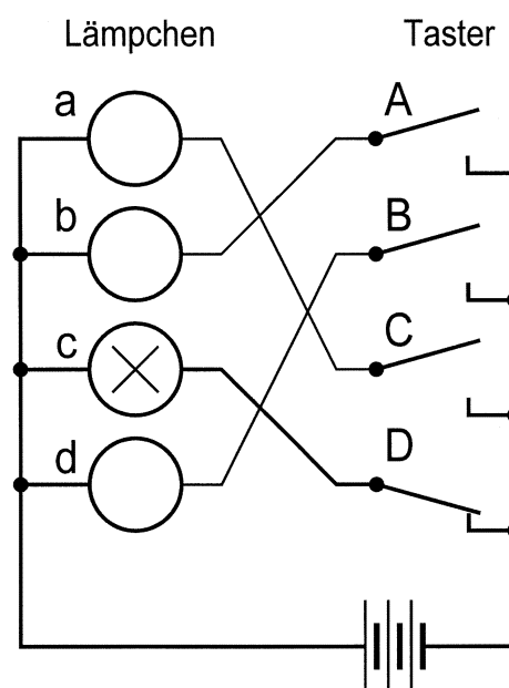
34 Eine monoalphabetische Verschlüsselung, realisiert mit Tastern und Lämpchen. Es sind nur 4 Einheiten gezeichnet, tatsächlich sind es deren 26. [AUT]
