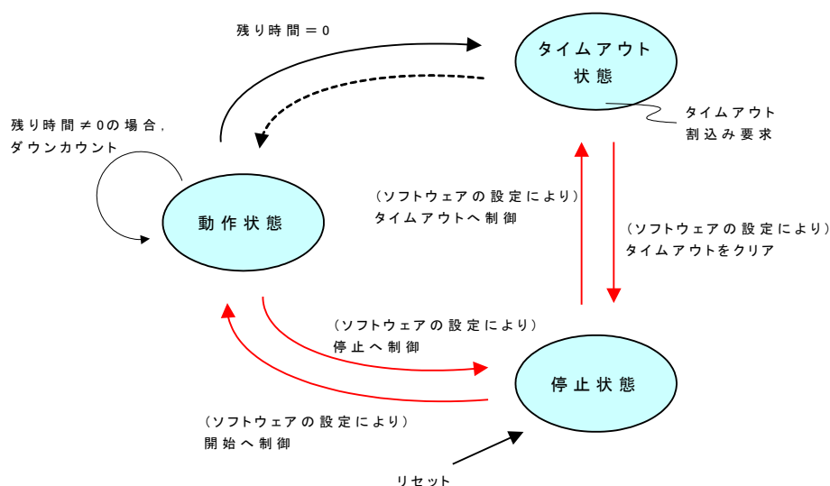
図 4-3 タイマの状態遷移の概念図
