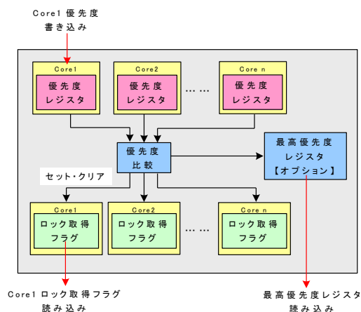
図 5-2 優先度順スピンロックユニットの概念モデル
