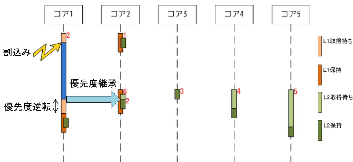
図 5-5 ネストロックにおける優先度継承
