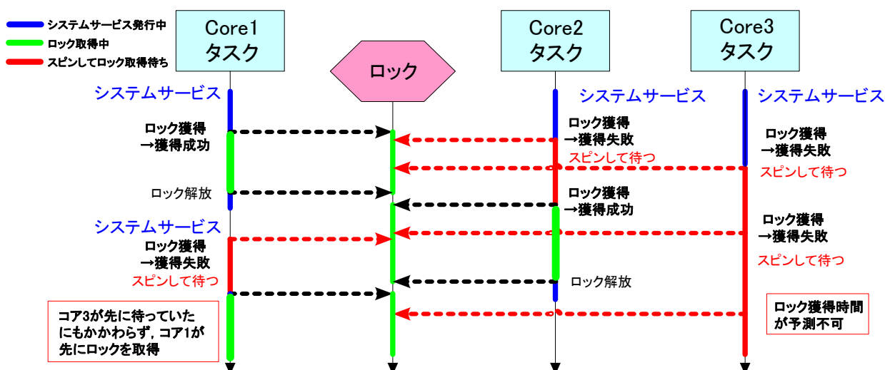
図 3-2 Test and Set スピンロックの問題点
