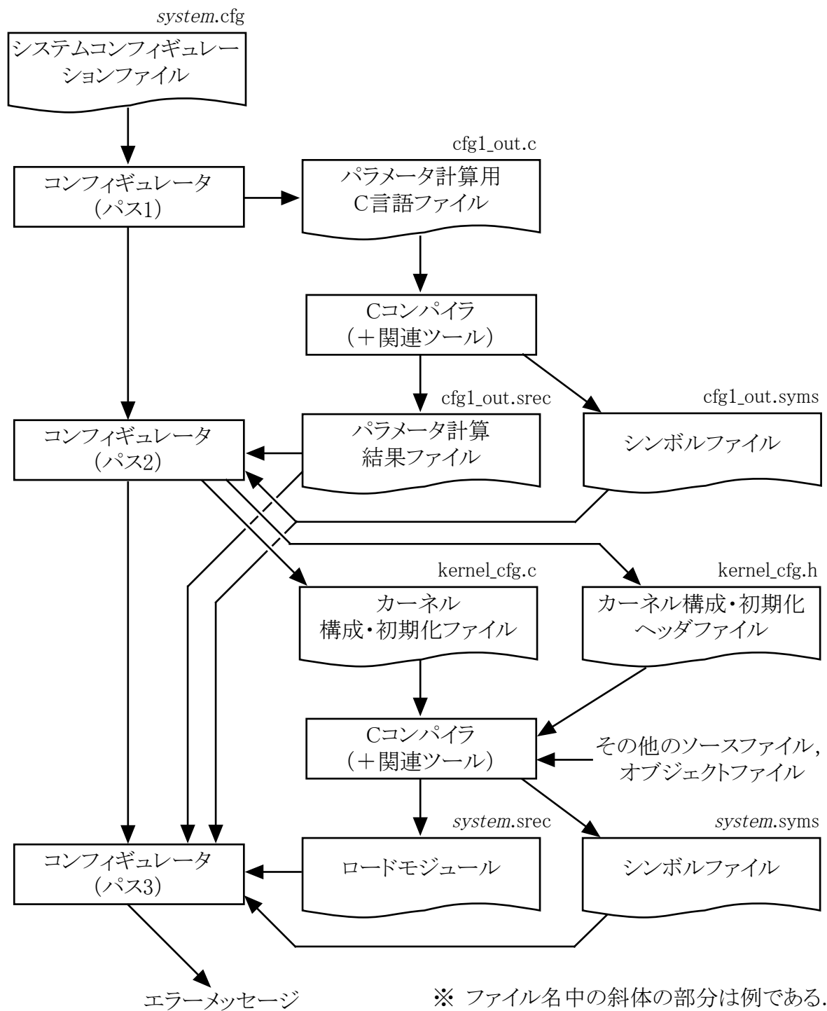
図2-10. コンフィギュレータの処理モデル
