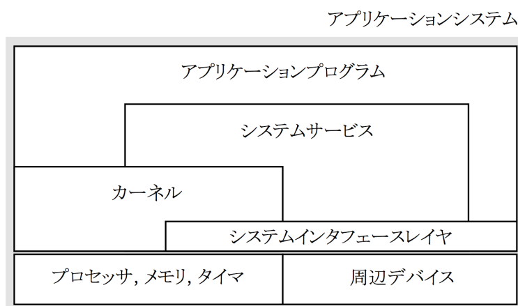
図2-1. 想定するソフトウェア構成
