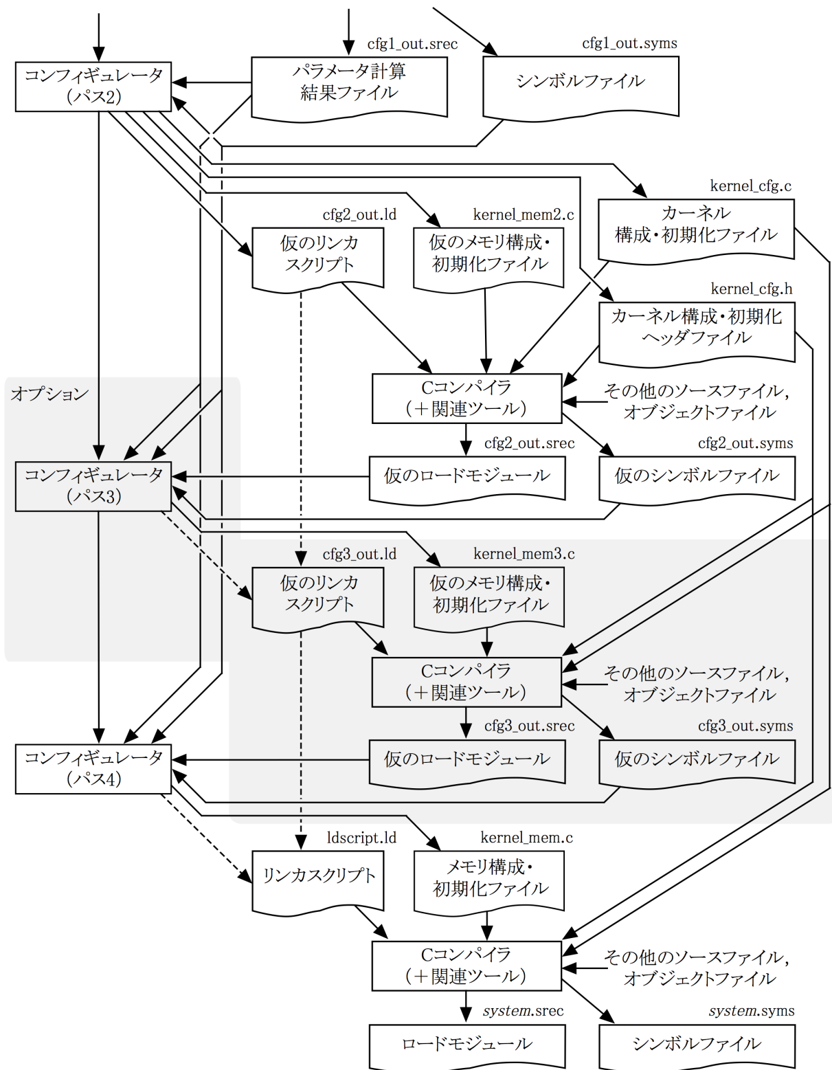
図2-11. 保護機能対応カーネルにおけるコンフィギュレータの処理モデル
