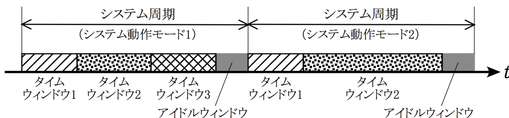
図2-4. システム周期毎のタイムウィンドウの実行
