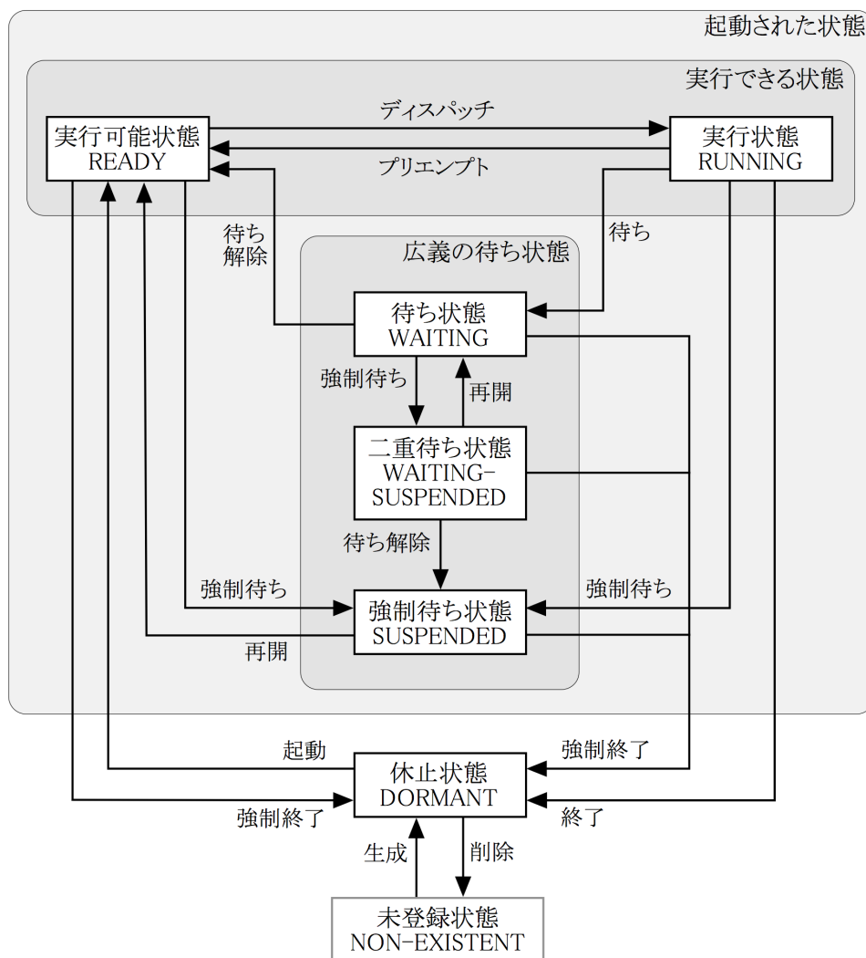
図2-2. タスクの状態遷移
