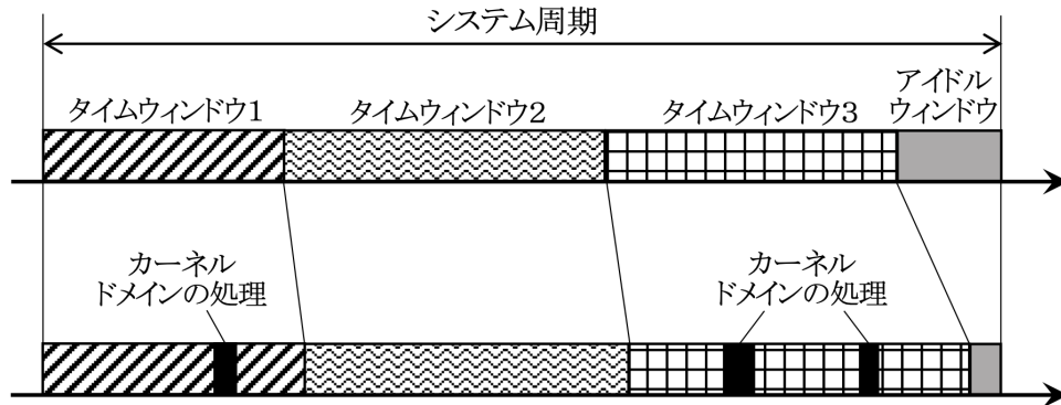
図2-5. タイムウィンドウの切換えタイミング
