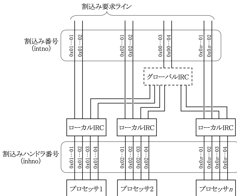
図2-7. マルチプロセッサ対応カーネルにおける割込み番号と割込みハンドラ番号
