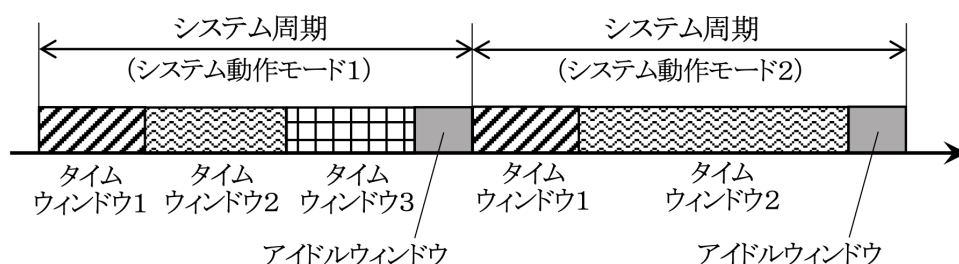
図2-4. システム周期毎のタイムウィンドウの実行
