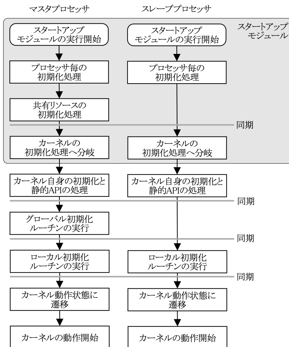
図2-8. マルチプロセッサ対応カーネルにおけるシステム初期化の流れ
