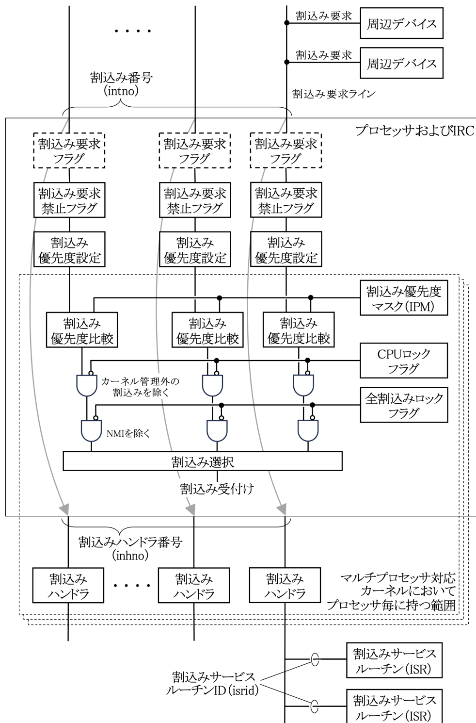
図2-6. TOPPERS標準割り込み処理モデルの概念図
